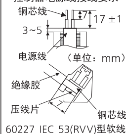
控制器电源线接线要求
