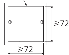
标准86型接线盒
