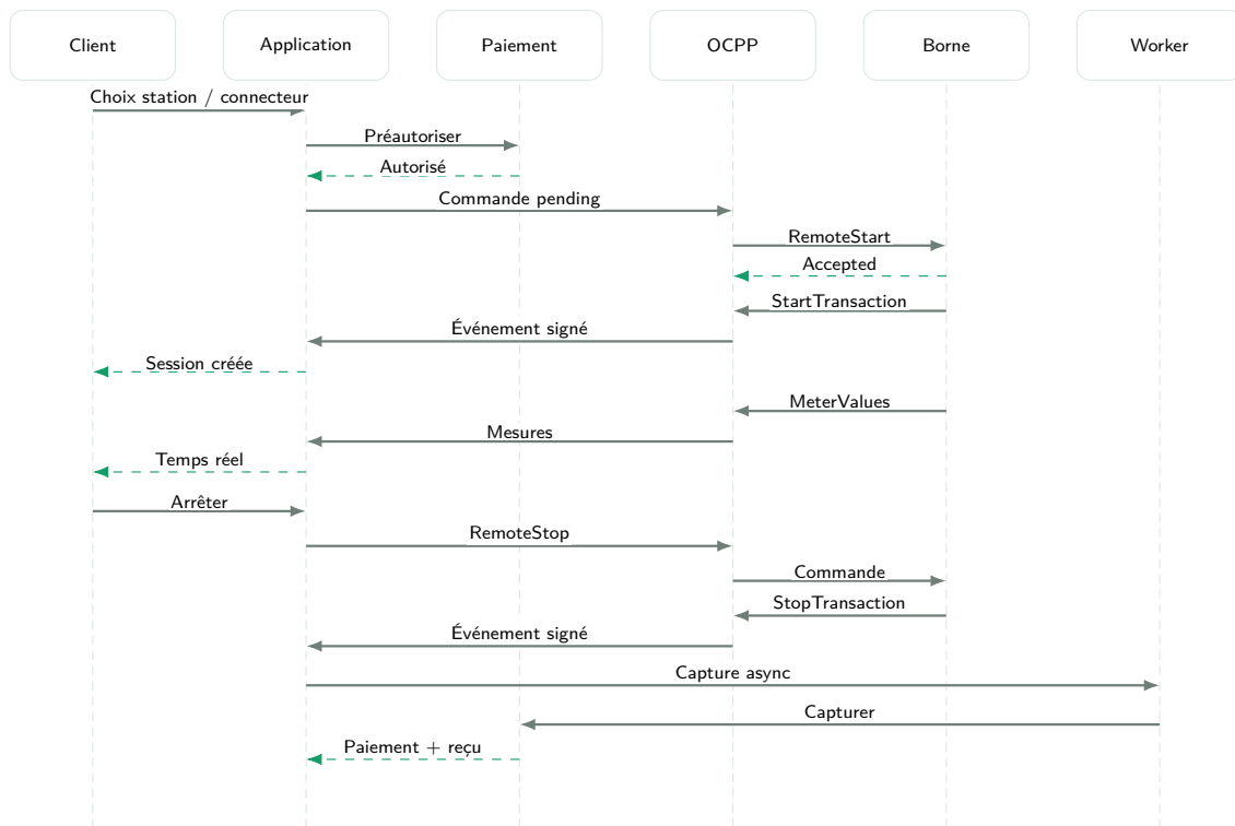
Figure 3.6 – Séquence de recharge distante et paiement simulé
