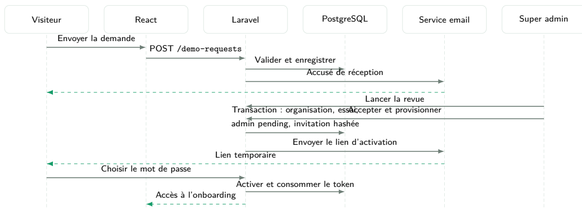
Figure 3.4 – Provisionnement d'une organisation à partir d'une demande de démonstration
