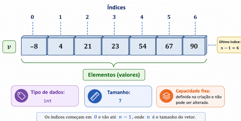
Figura 9.1. Estrutura de um vetor (array) unidimensional com índices e elementos.
