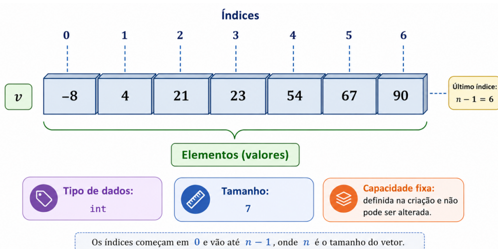
Figura 8.1. Estrutura de um vetor (array) unidimensional com índices e elementos.
