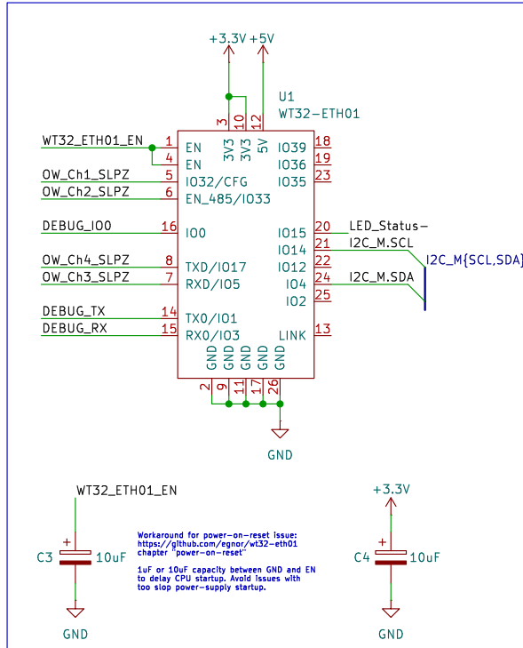
MCU: WT32-ETH01
