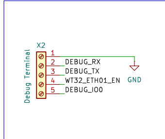
MCU: WT32-ETH01
