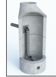
Beispiel: FUNKE I.A. innenliegender Abfluss
