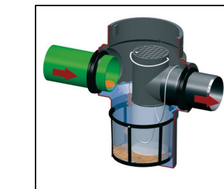
Beispiel: PREMIER TECH Rewatec Vorflut Masi Plus
