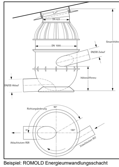
Beispiel: ROMOLD Energieumwandlungsschacht
