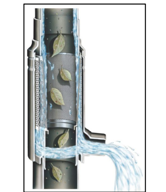
Beispiel: WSV Filtersammel FS
