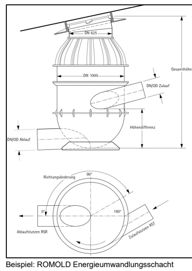
Beispiel: ROMOLD Energieumwandlungsschacht
