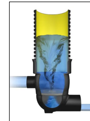
Beispiel: FRANKISCHE Rigo Limit V
