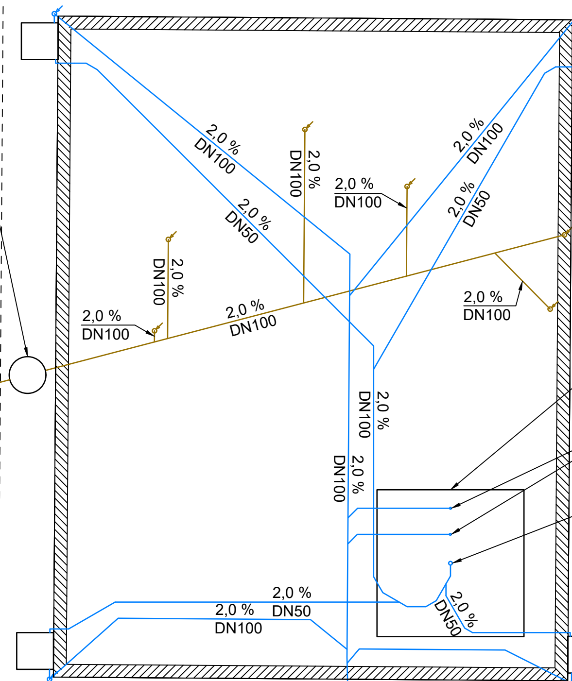
Beispiel: FUNKE I.A. innenliegender Absturz
