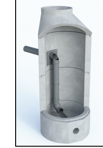
Beispiel: FUNKE I.A. innenliegender Absturz
