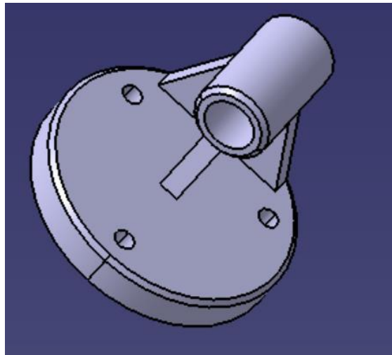
Figure 5: Support de montage — modélisation réalisée sous CATIA V5.
