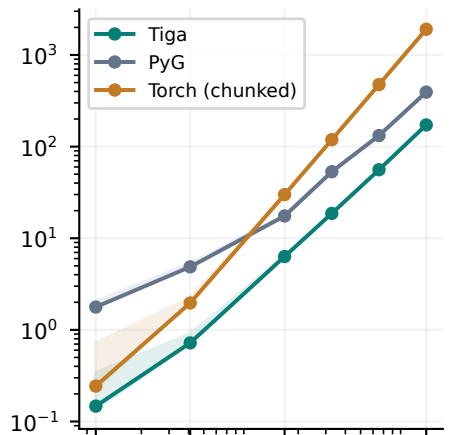
Dynamic exact kNN · F=1
