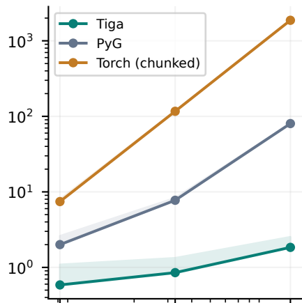
Dynamic radius · F=1
