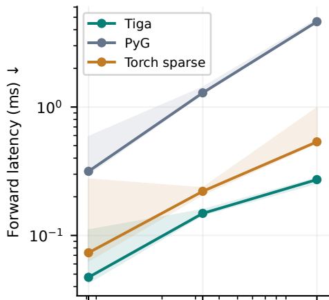
Stored CSR · F=32
