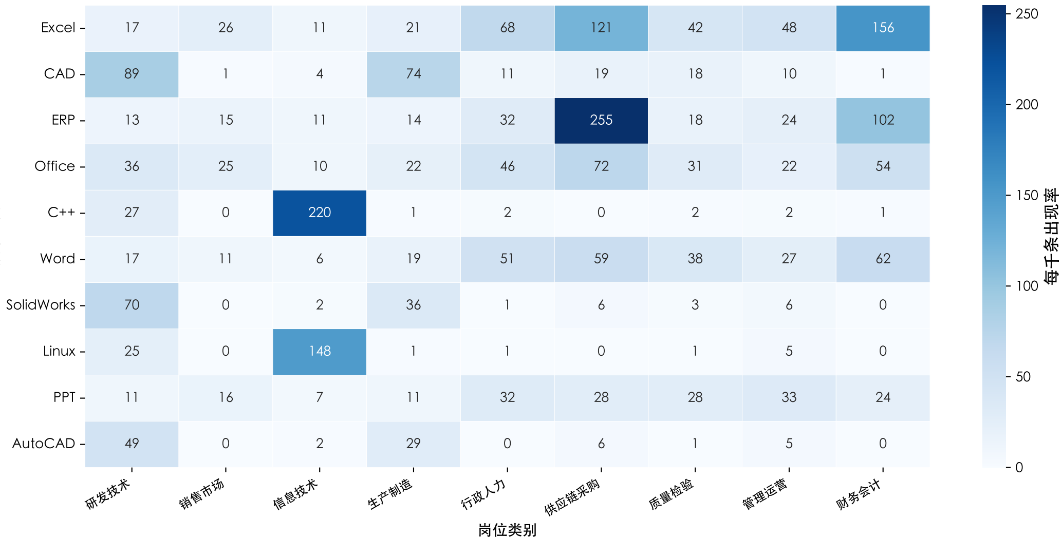
各岗位类别技术工具需求热力图（每千条出现率）
