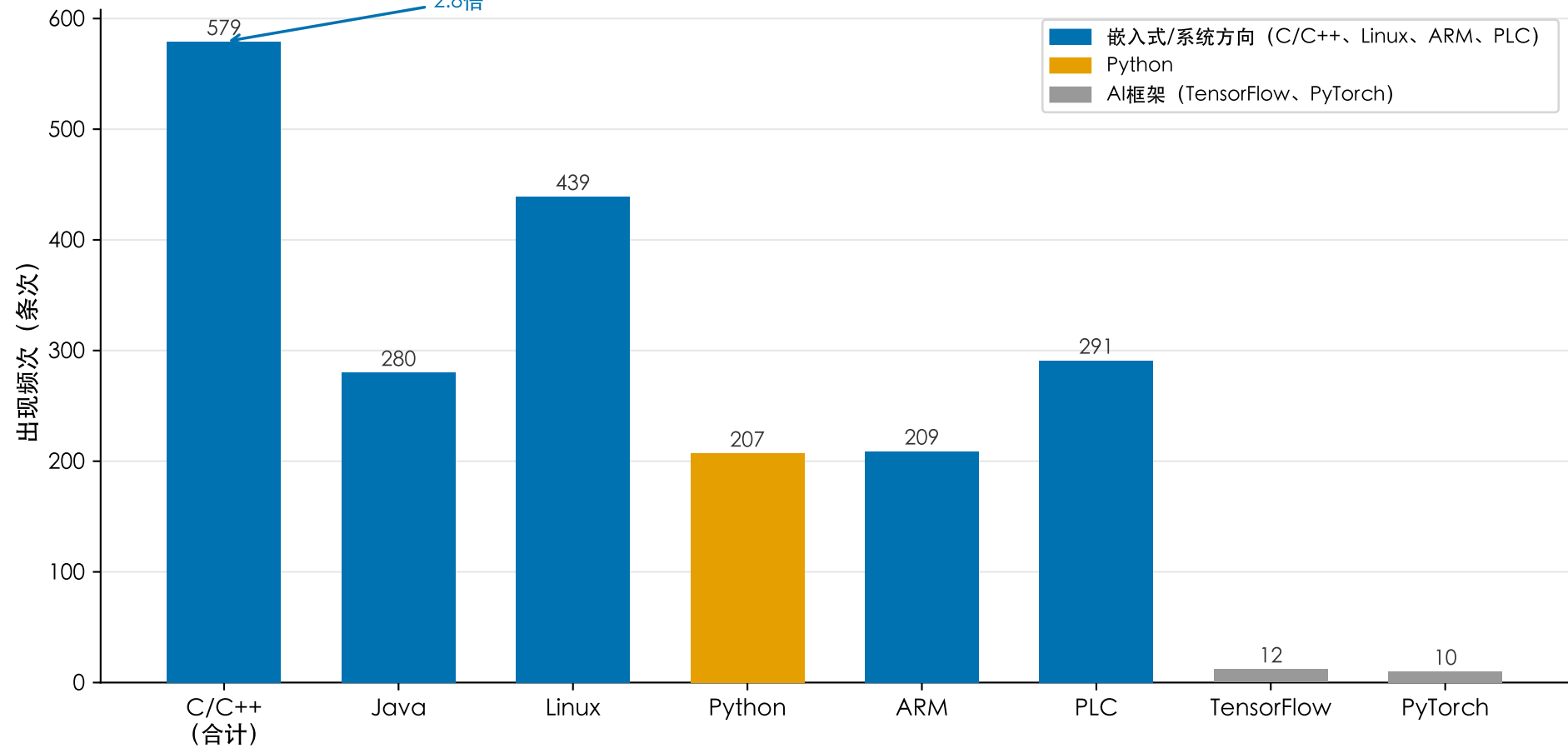
C/C++编程/系统工具频次对比：嵌入式方向 vs Python vs AI框架
