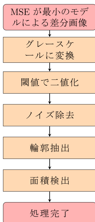
Figure 1.14: 差分画像の処理フロー
