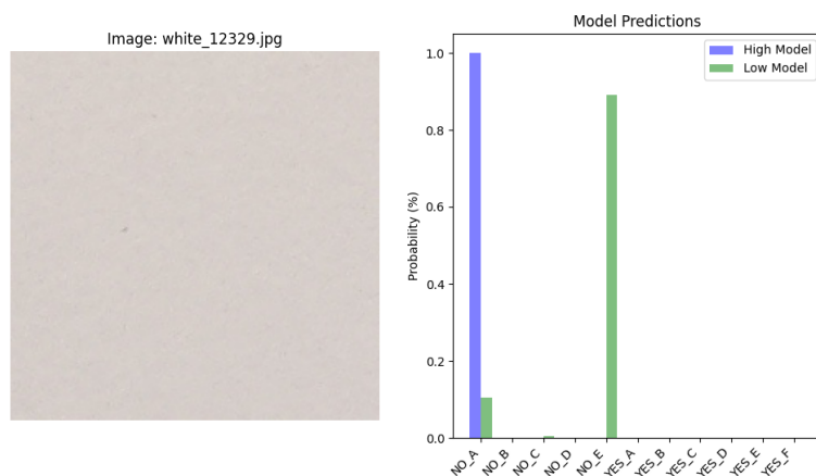
図 1.11: テスト画像 1 の予測結果
