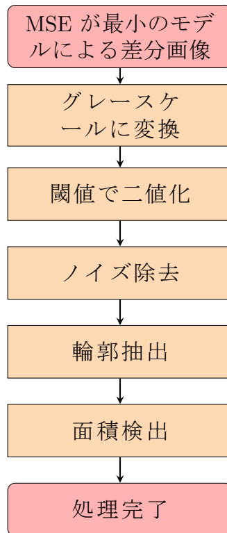
図 1.14: 差分画像の処理フロー
