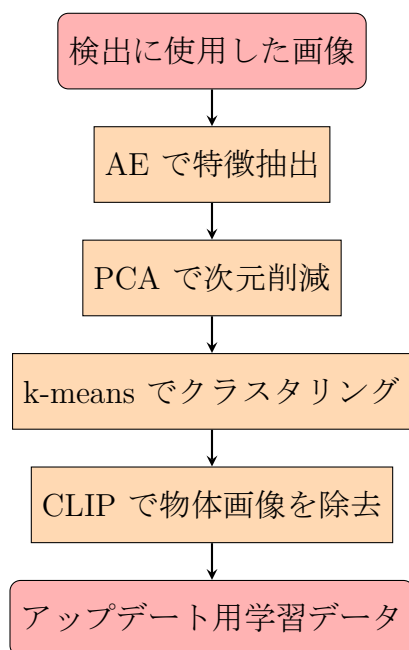
図 1.6: モデルのアップデート方法の流れ
