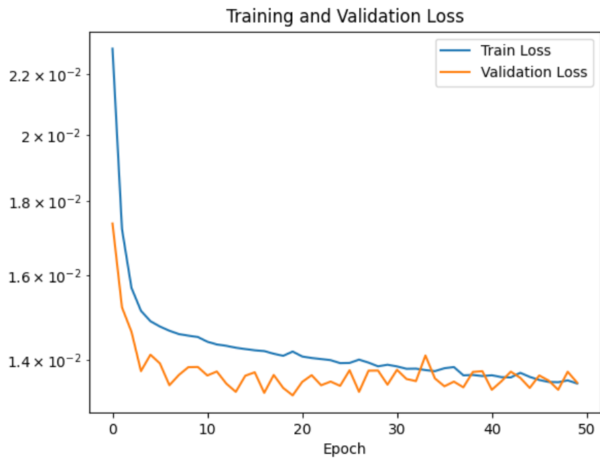
図 1.65: 学習曲線
