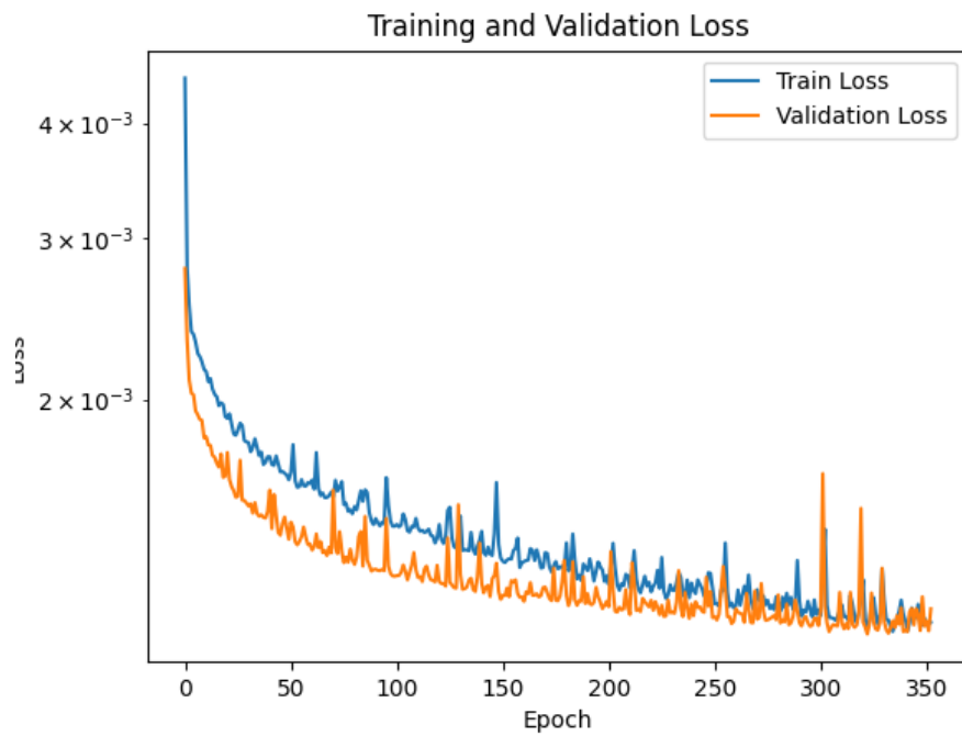
図 1.45: 学習曲線
