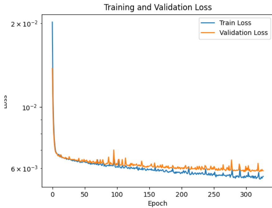
図 1.43: 学習曲線
