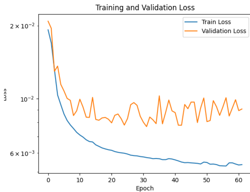
図 1.72: 学習曲線
