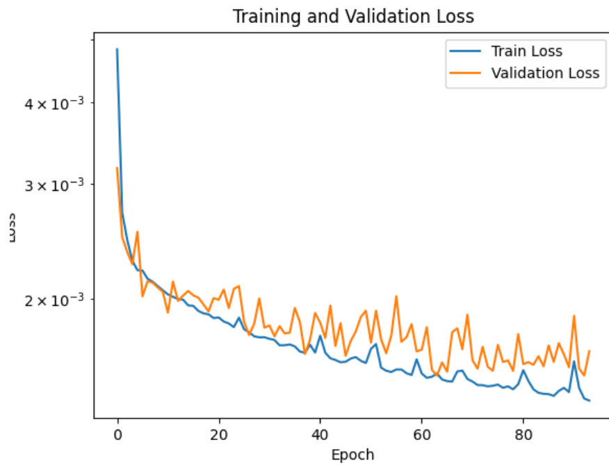
図 1.63: 学習曲線
