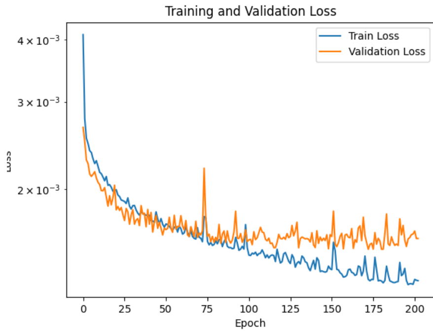
図 1.56: 学習曲線
