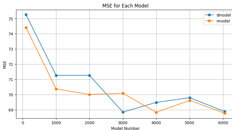
図 1.23: MSE の推移
