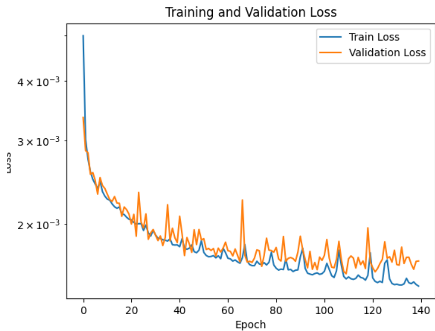
図 1.50: 学習曲線
