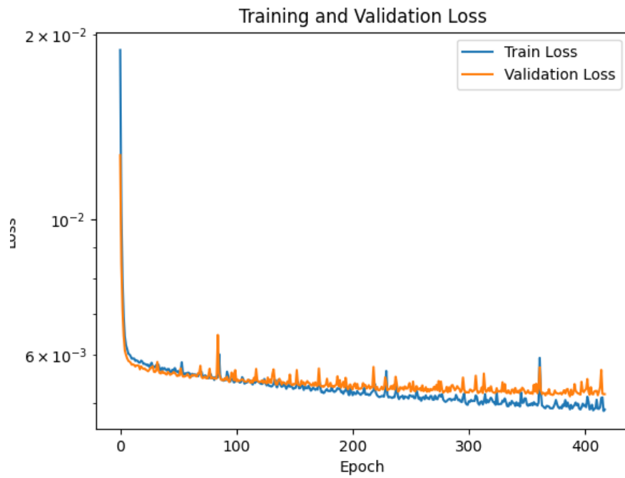
図 1.42: 学習曲線
