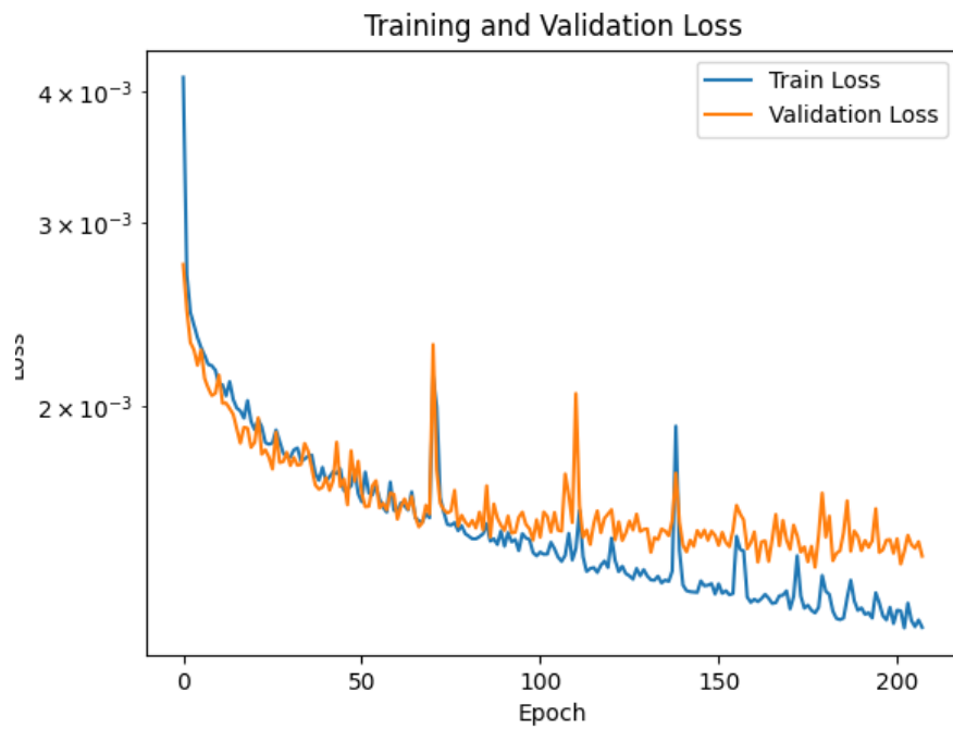
図 1.57: 学習曲線
