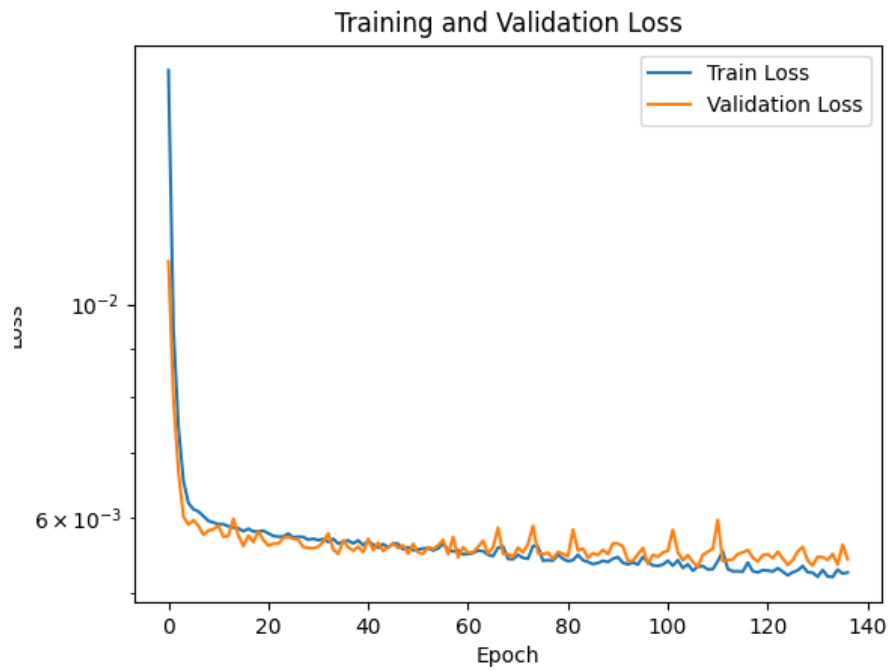
図 1.54: 学習曲線
