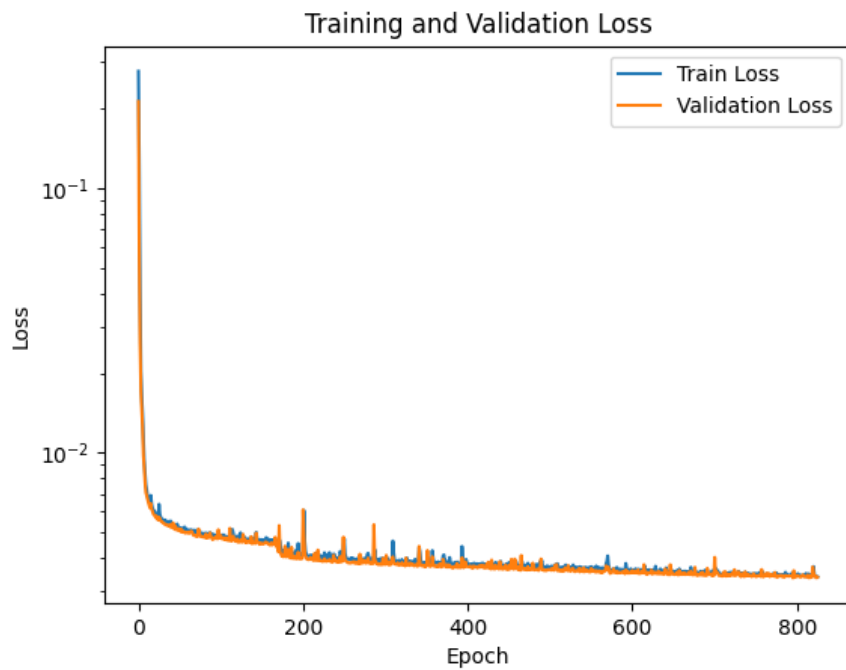
図 1.26: 学習曲線
