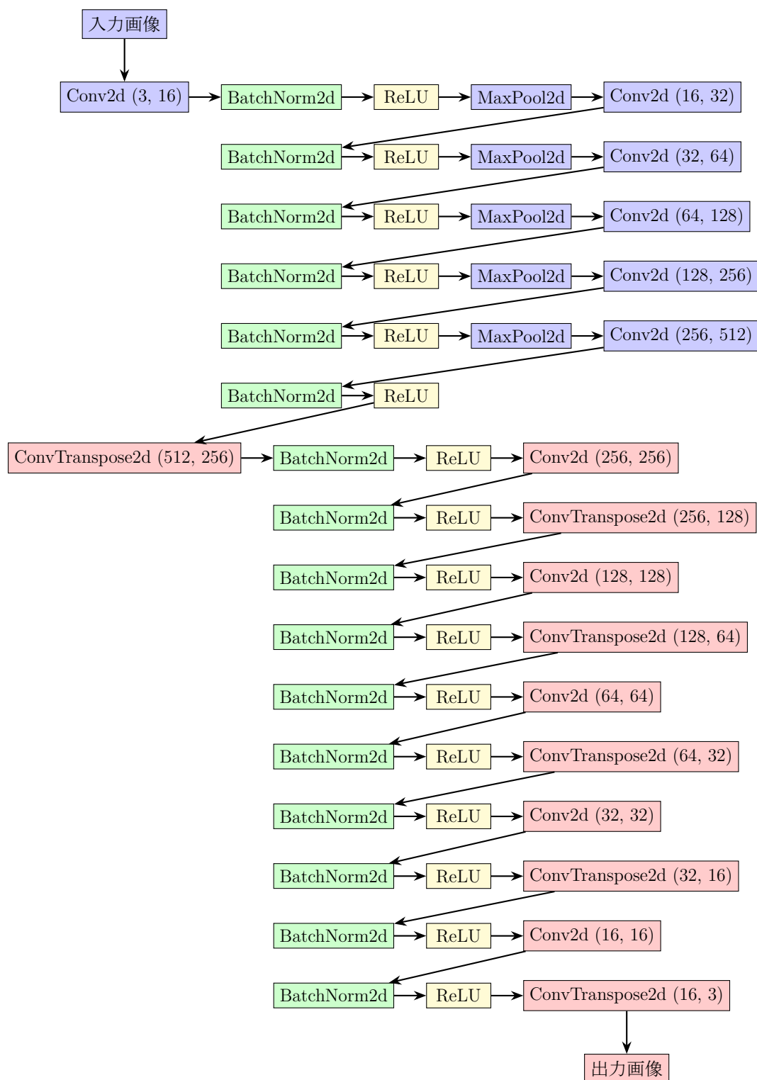
図 1.4: AE の構造
