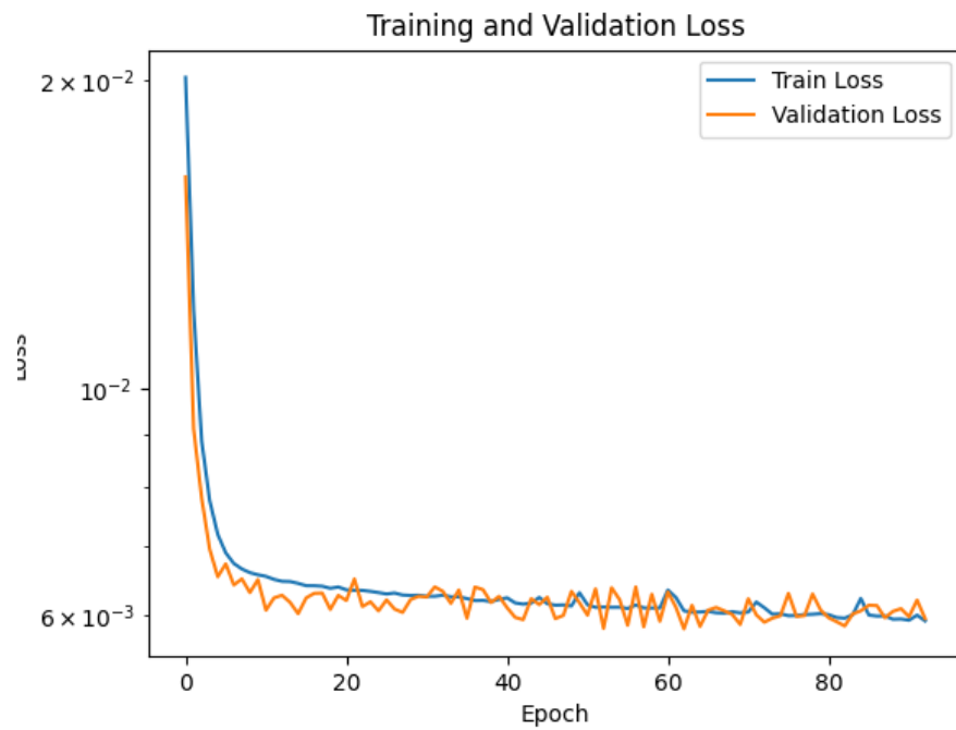
図 1.61: 学習曲線
