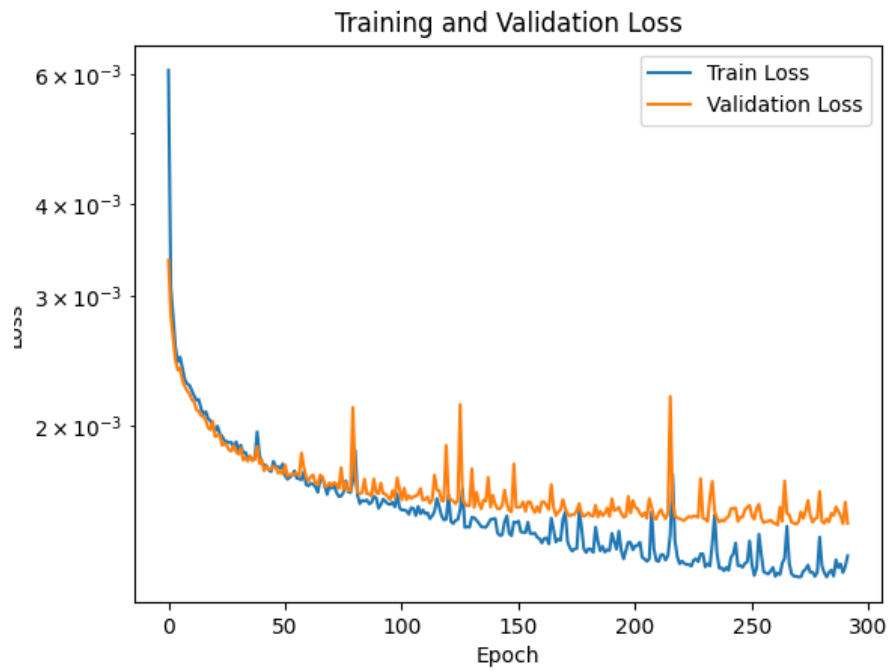
図 1.44: 学習曲線
