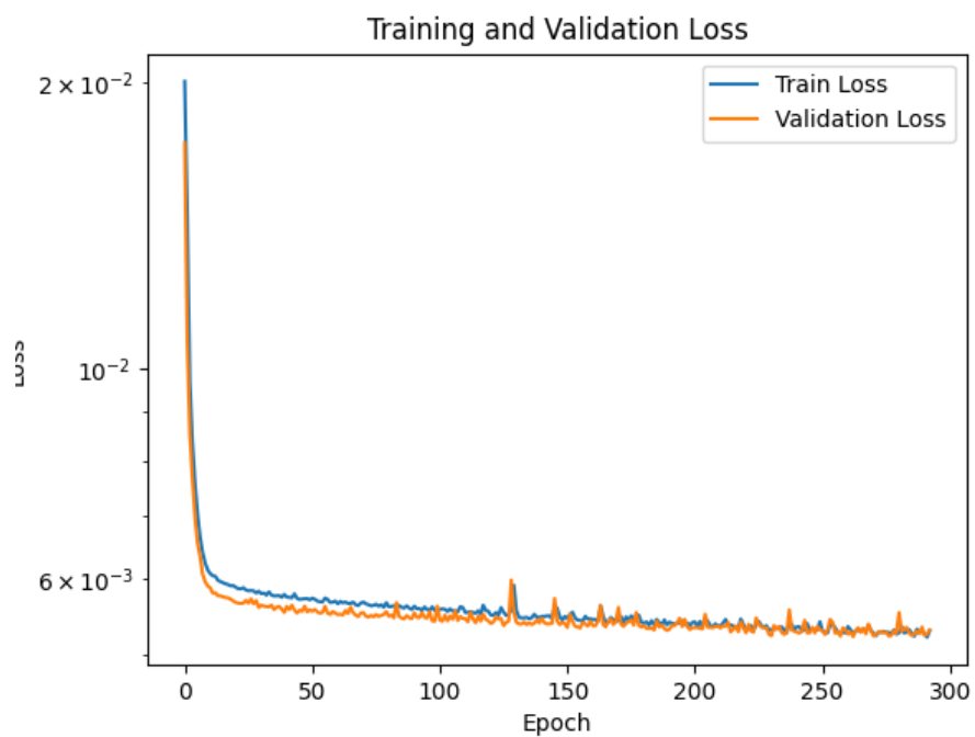
図 1.36: 学習曲線
