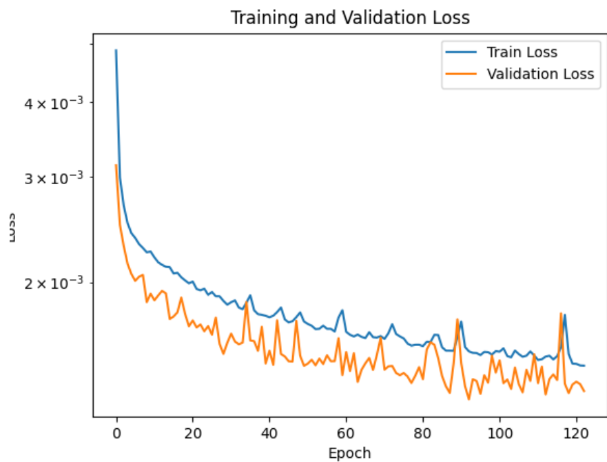
図 1.51: 学習曲線
