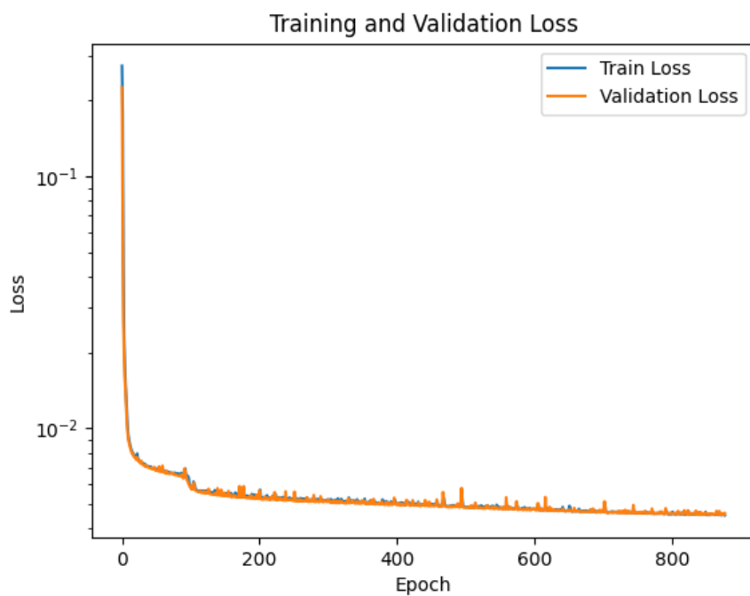
図 1.28: 学習曲線
