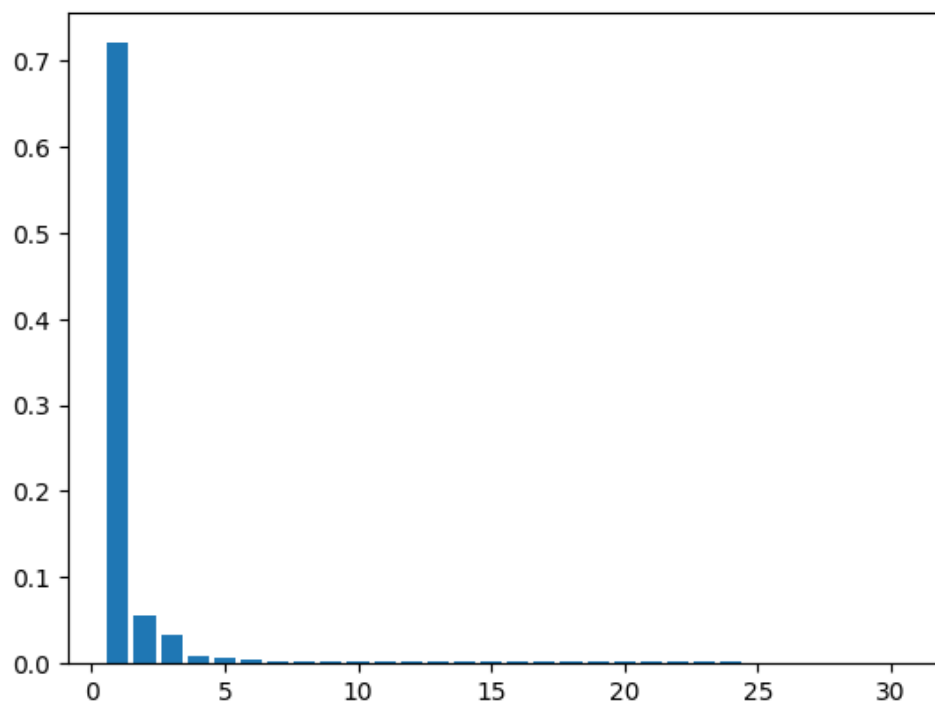
図 1.7: 主成分分析の寄与度
