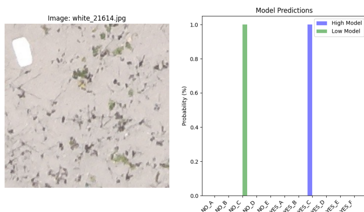
図 1.12: テスト画像 2 の予測結果
