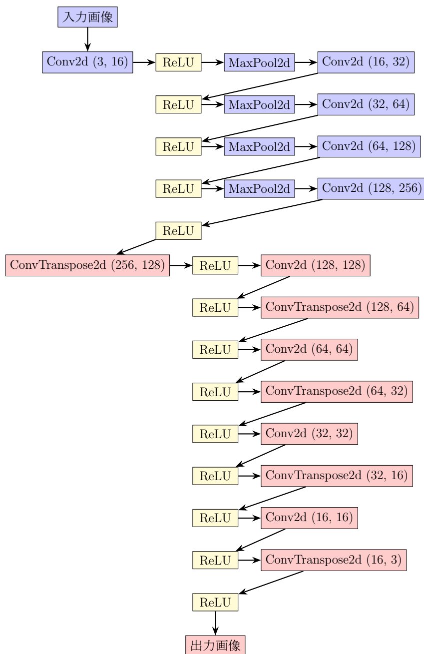
図 1.5: 今年度の AE の構造
