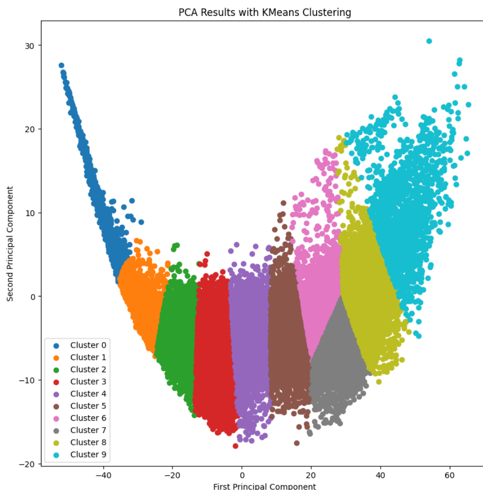
図 1.10: k-means クラスタリングの結果
