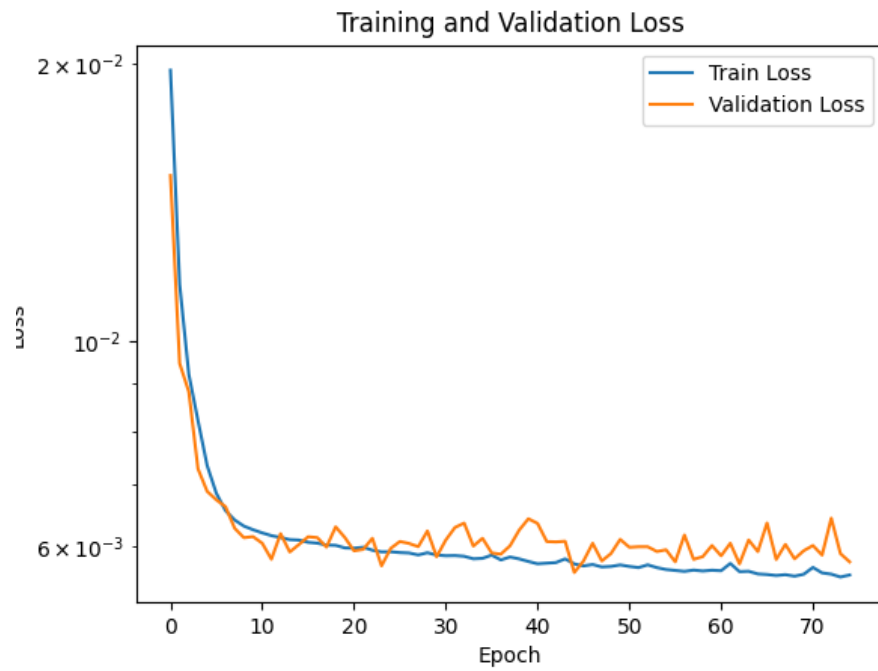
図 1.66: 学習曲線
