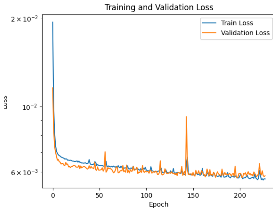
図 1.55: 学習曲線
