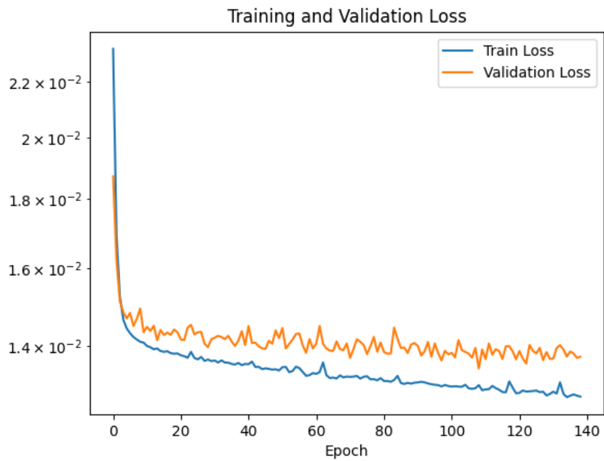
図 1.47: 学習曲線
