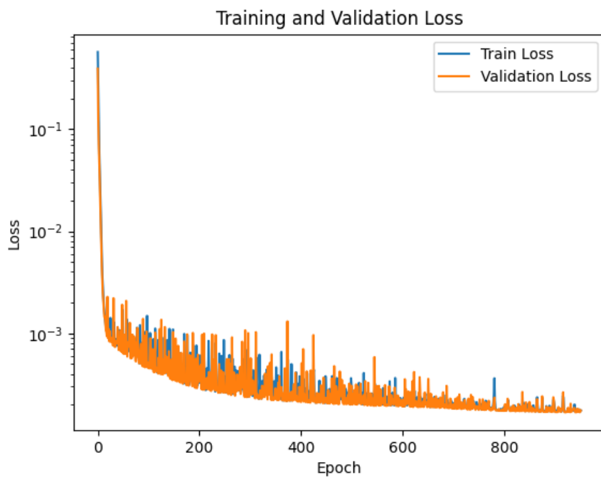
図 1.29: 学習曲線
