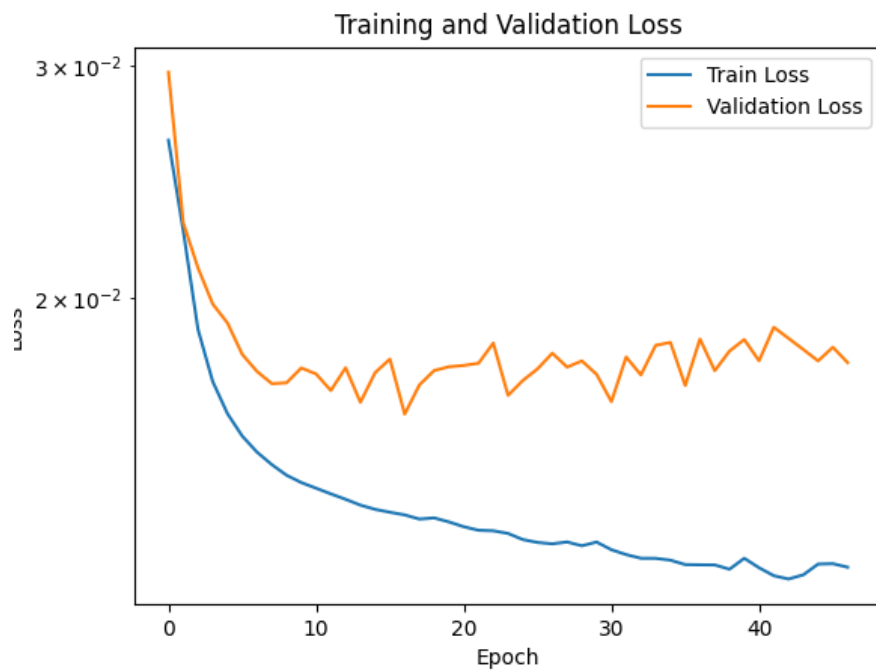
図 1.70: 学習曲線
