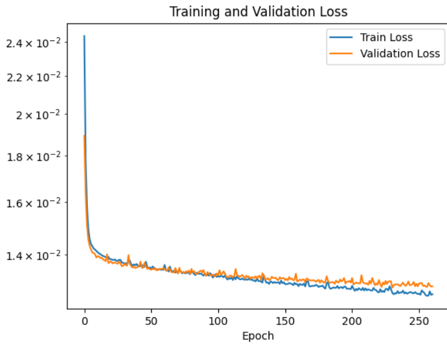
図 1.30: 学習曲線
