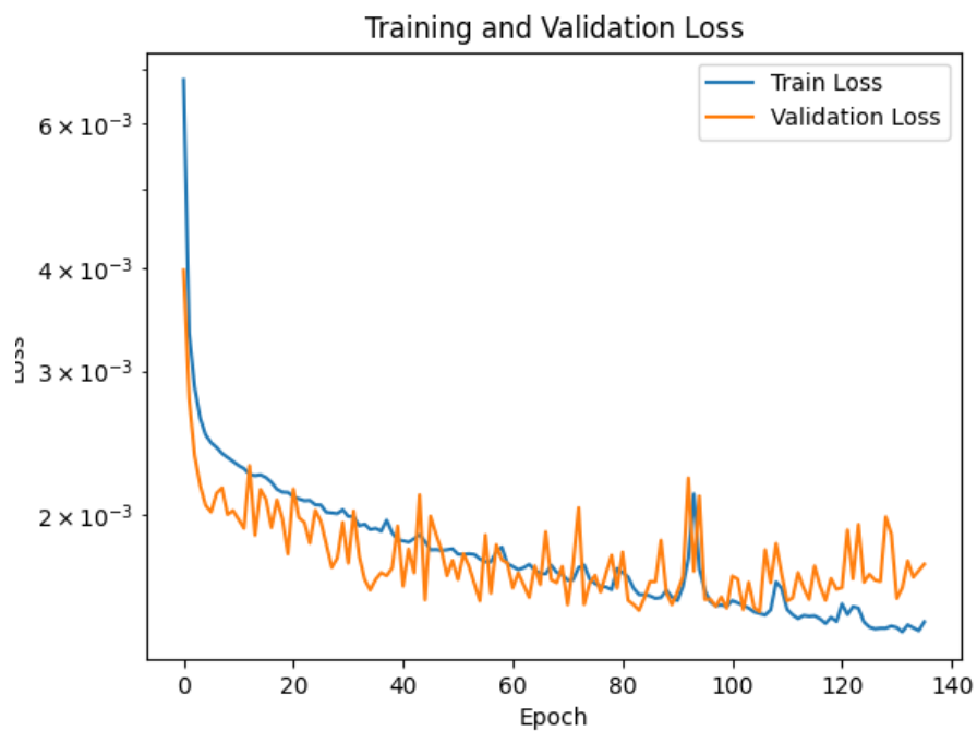
図 1.69: 学習曲線
