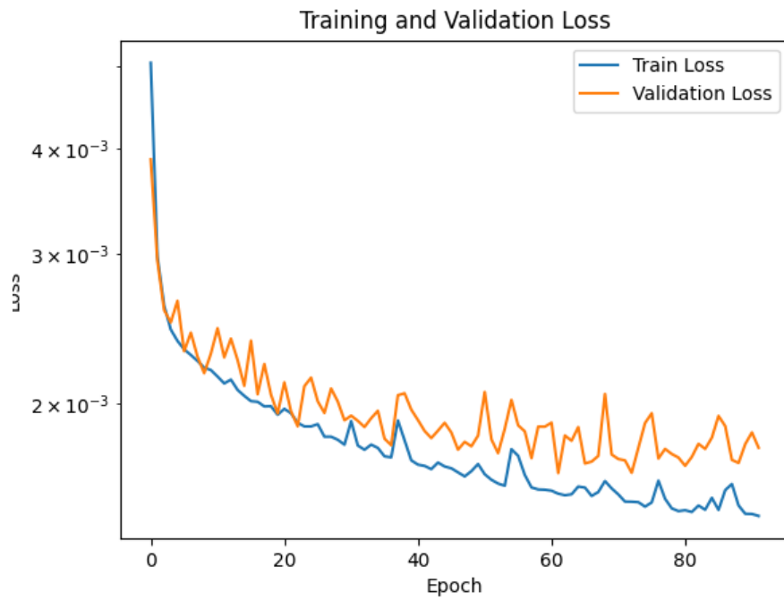
図 1.62: 学習曲線
