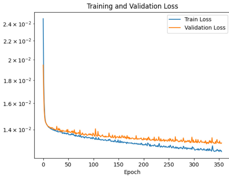
図 1.33: 学習曲線
