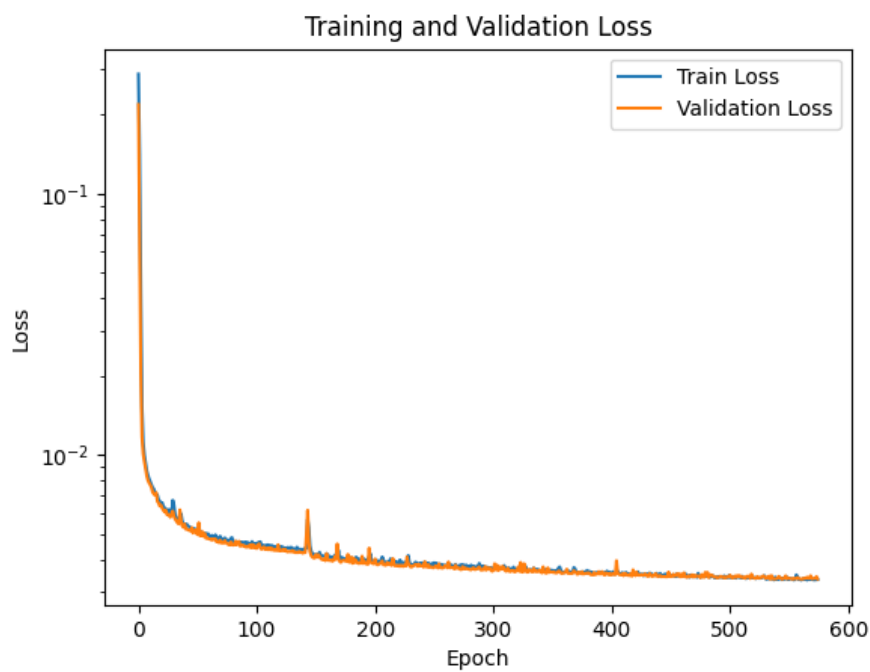
図 1.27: 学習曲線
