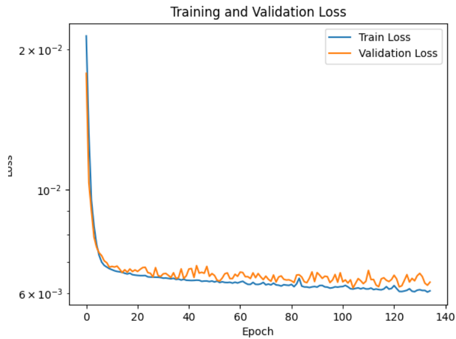
図 1.49: 学習曲線
