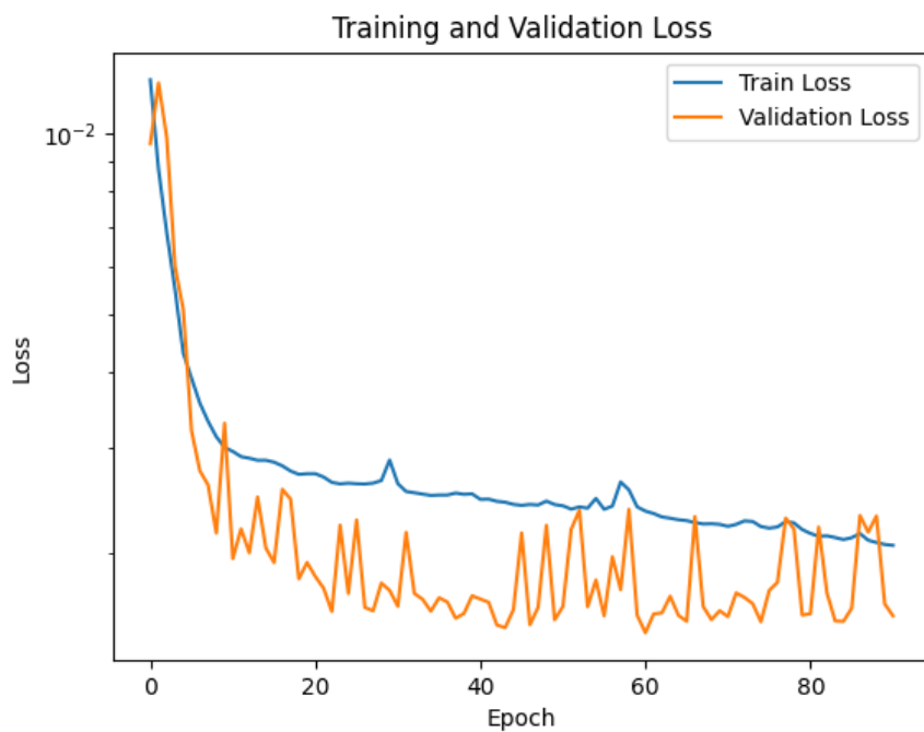
図 1.75: 学習曲線
