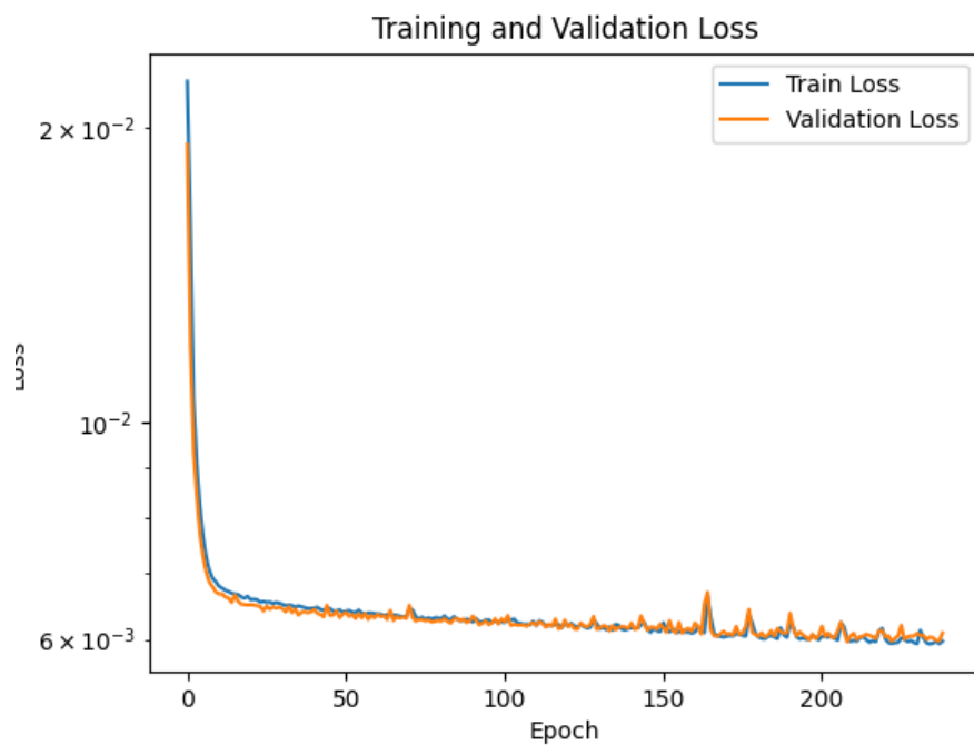
図 1.37: 学習曲線
