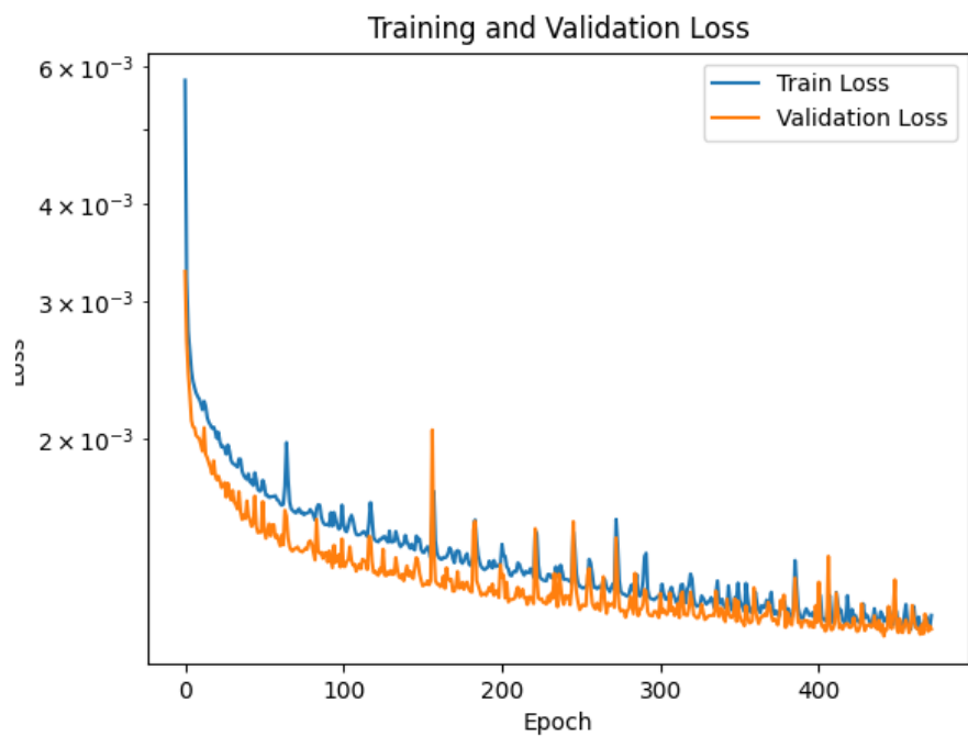
図 1.39: 学習曲線
