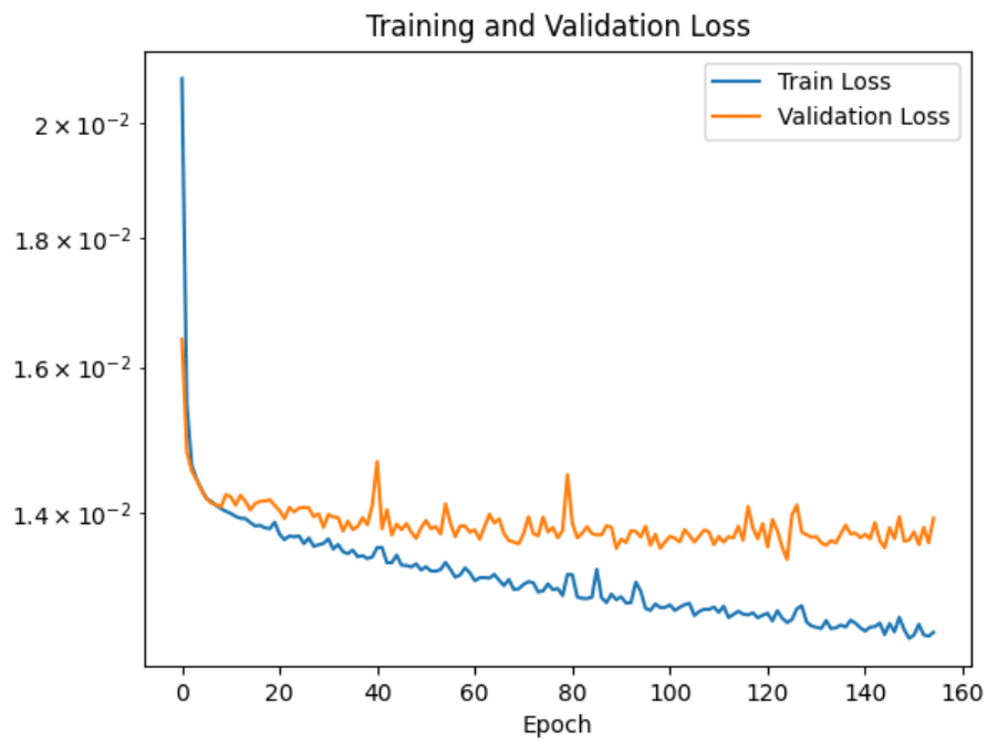
図 1.53: 学習曲線
