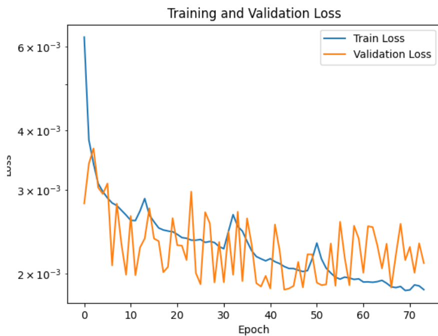
図 1.74: 学習曲線
