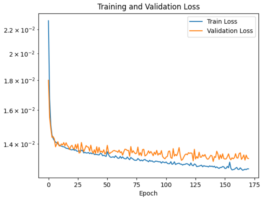
図 1.46: 学習曲線
