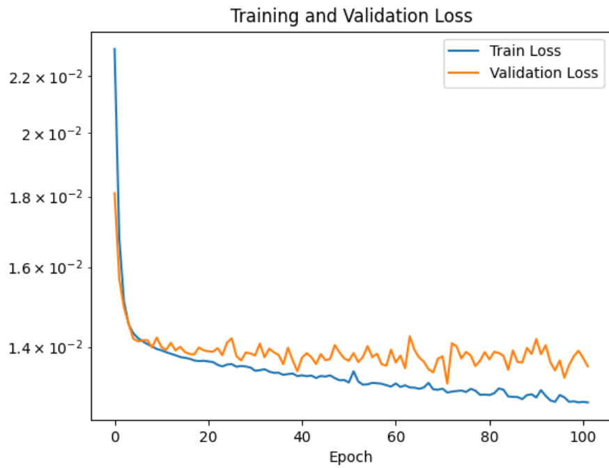
図 1.58: 学習曲線
