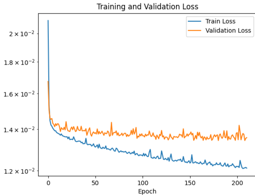
図 1.52: 学習曲線
