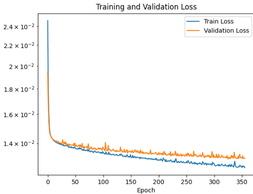
図 6.8: 学習曲線
