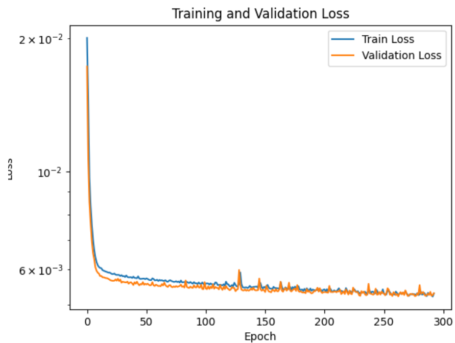
図 6.11: 学習曲線
