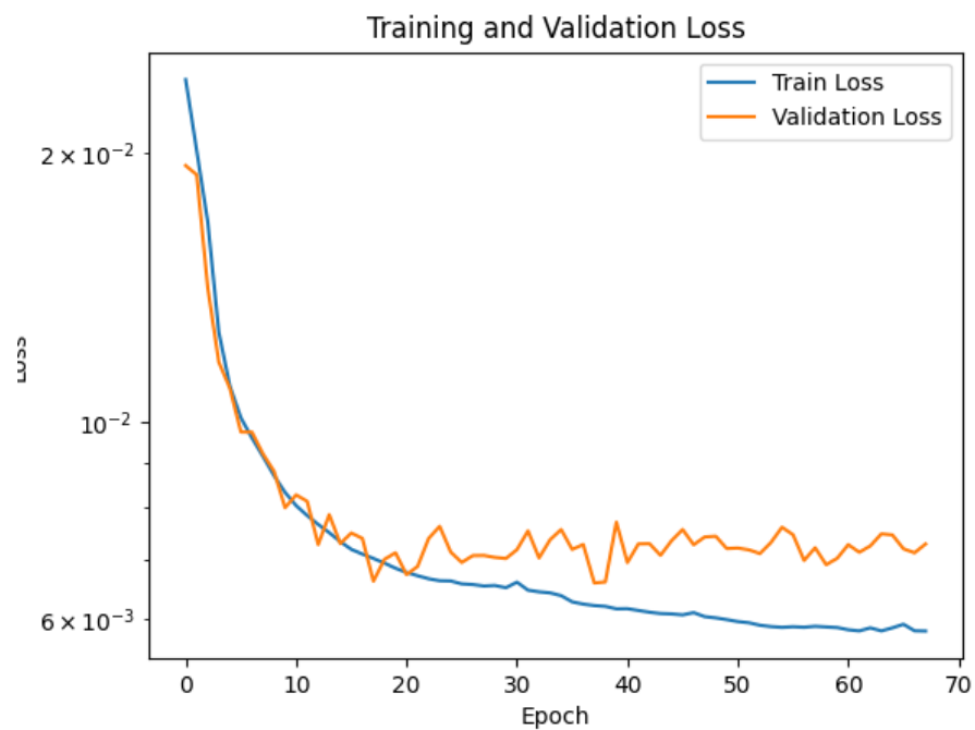
図 6.48: 学習曲線
