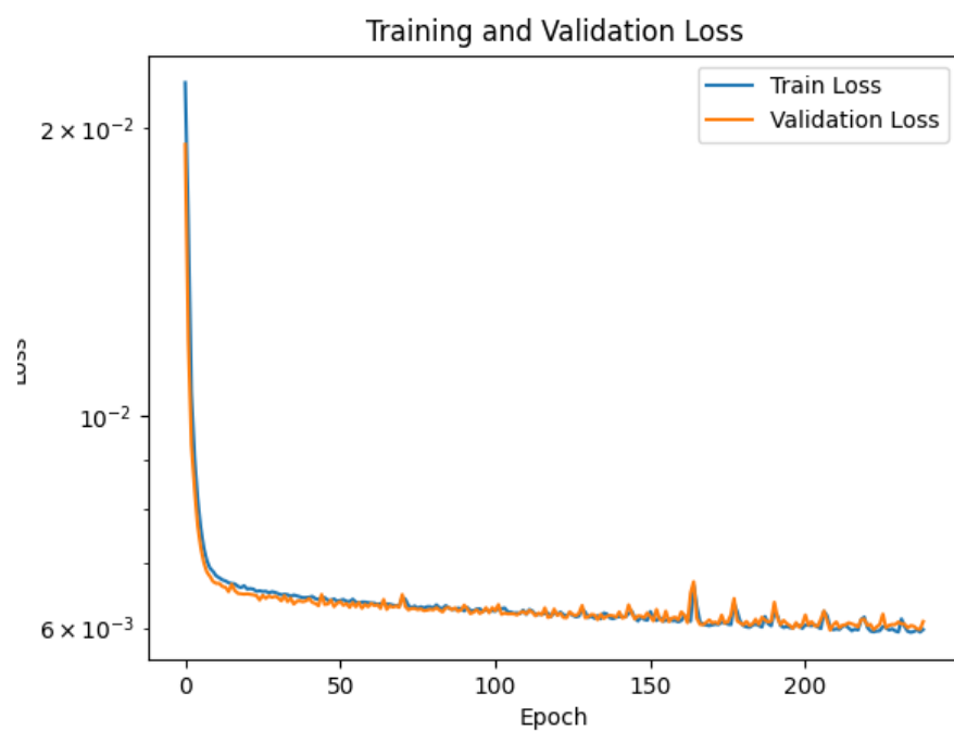
図 6.12: 学習曲線
