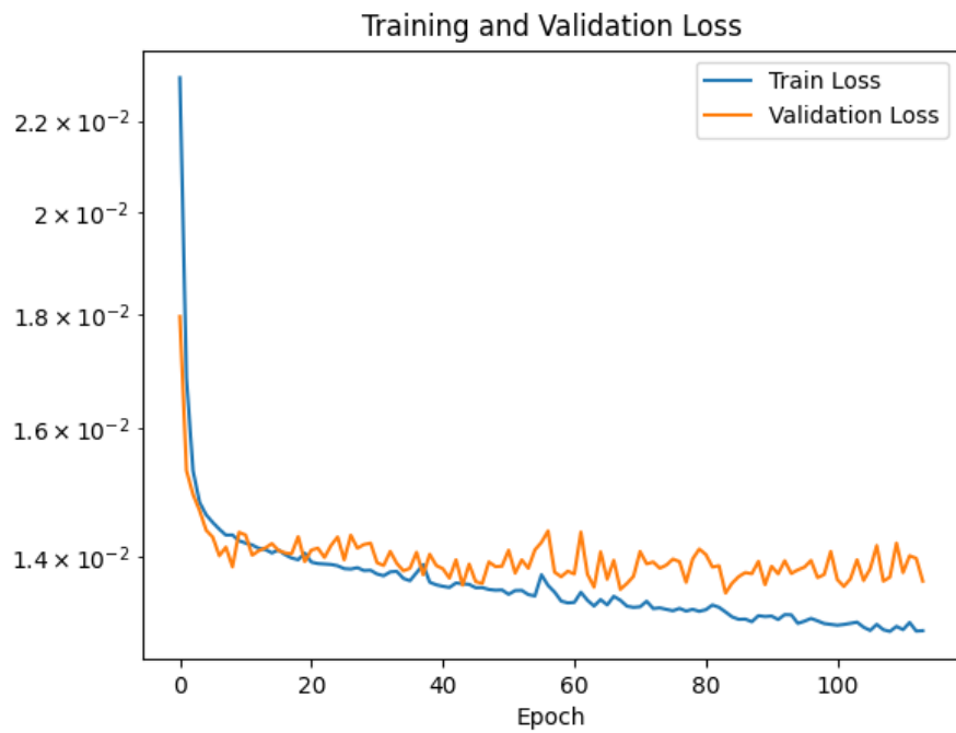
図 6.34: 学習曲線
