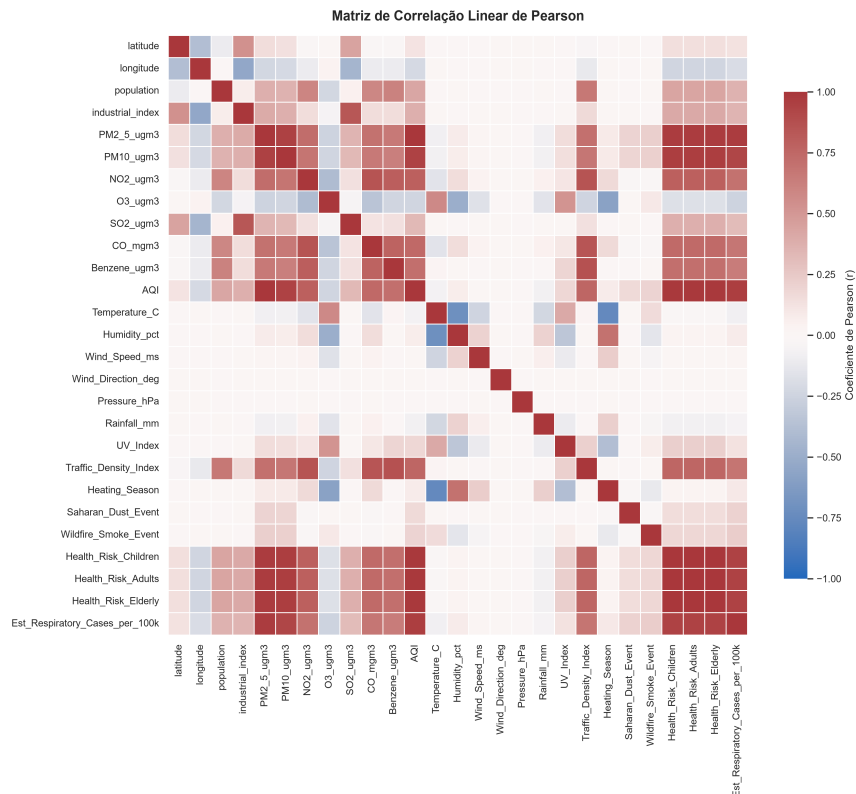
Figura 3: Matriz de correlação linear de Pearson para as 27 variáveis numéricas.
