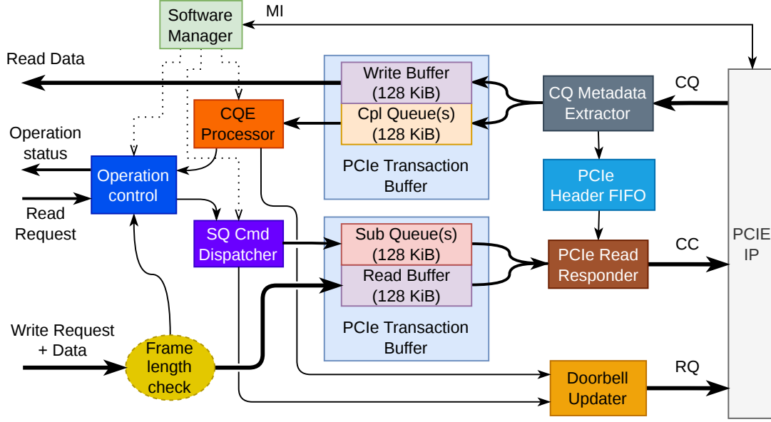
Fig. 4.6: DMA Iuventus block scheme
