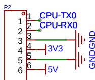
UART0
