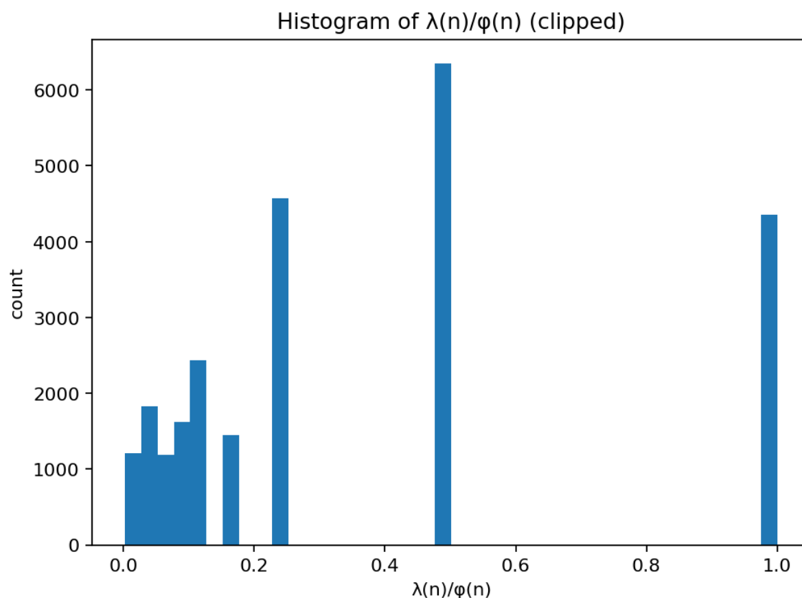
Fig. 19: E100 — Carmichael (n) vs. Euler (n)
