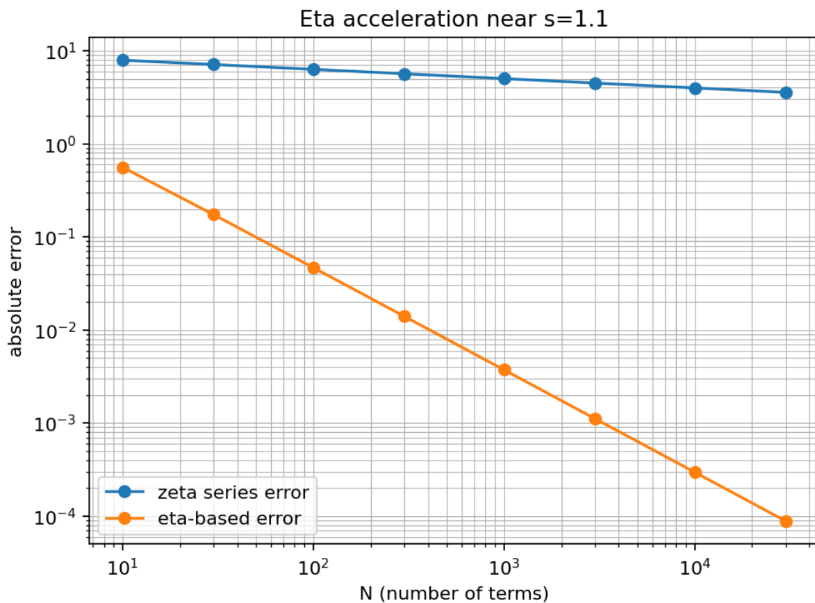
Fig. 4: E085 — Dirichlet eta acceleration for (s)
