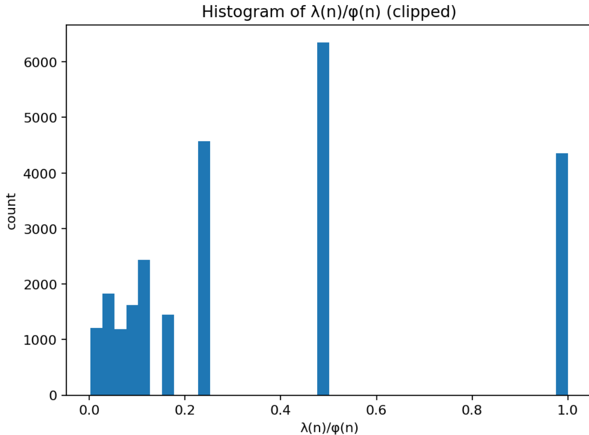
Fig. 19: E100 — Carmichael \lambda(n) vs. Euler \phi(n)
