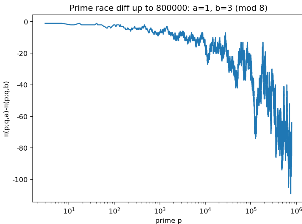
Fig. 32: E112 — Prime race: (x;q,a) - (x;q,b)
