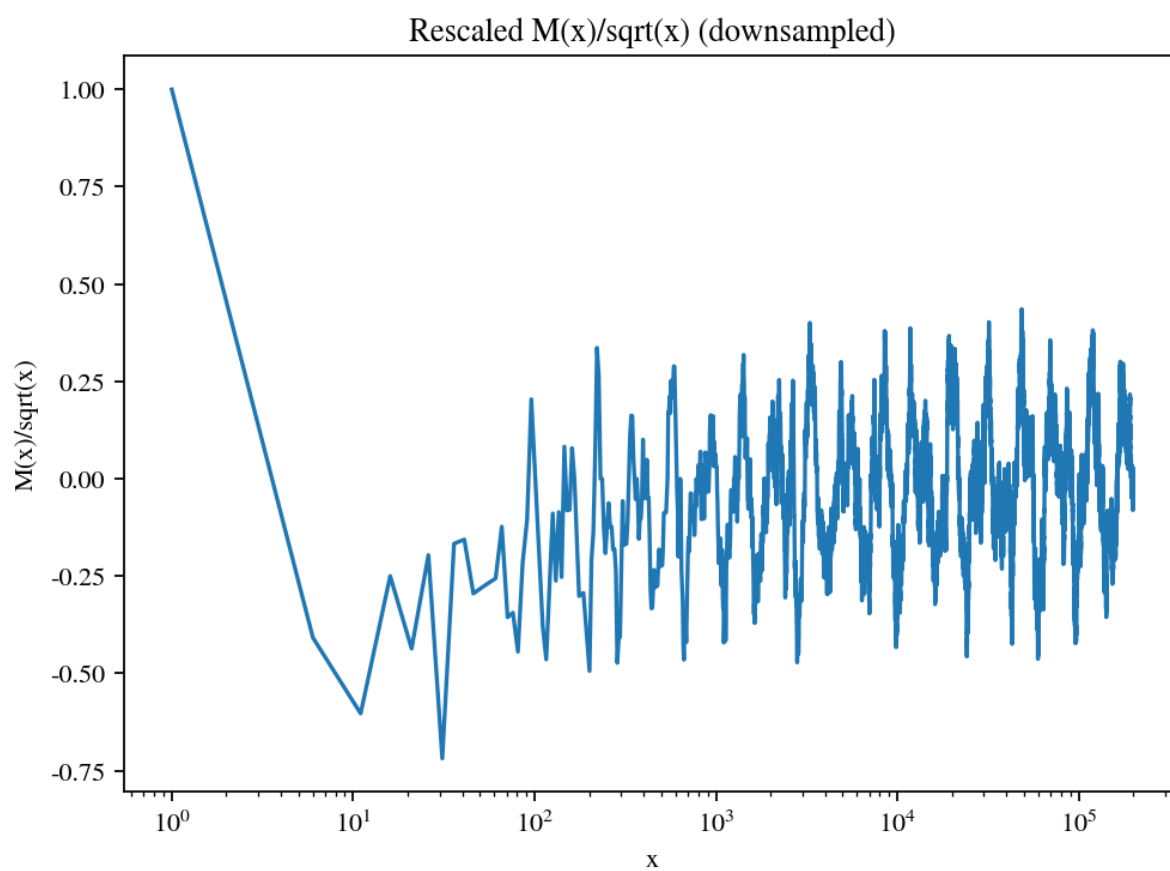
Fig. 25: E105 — Mertens M(x) : scaling views
