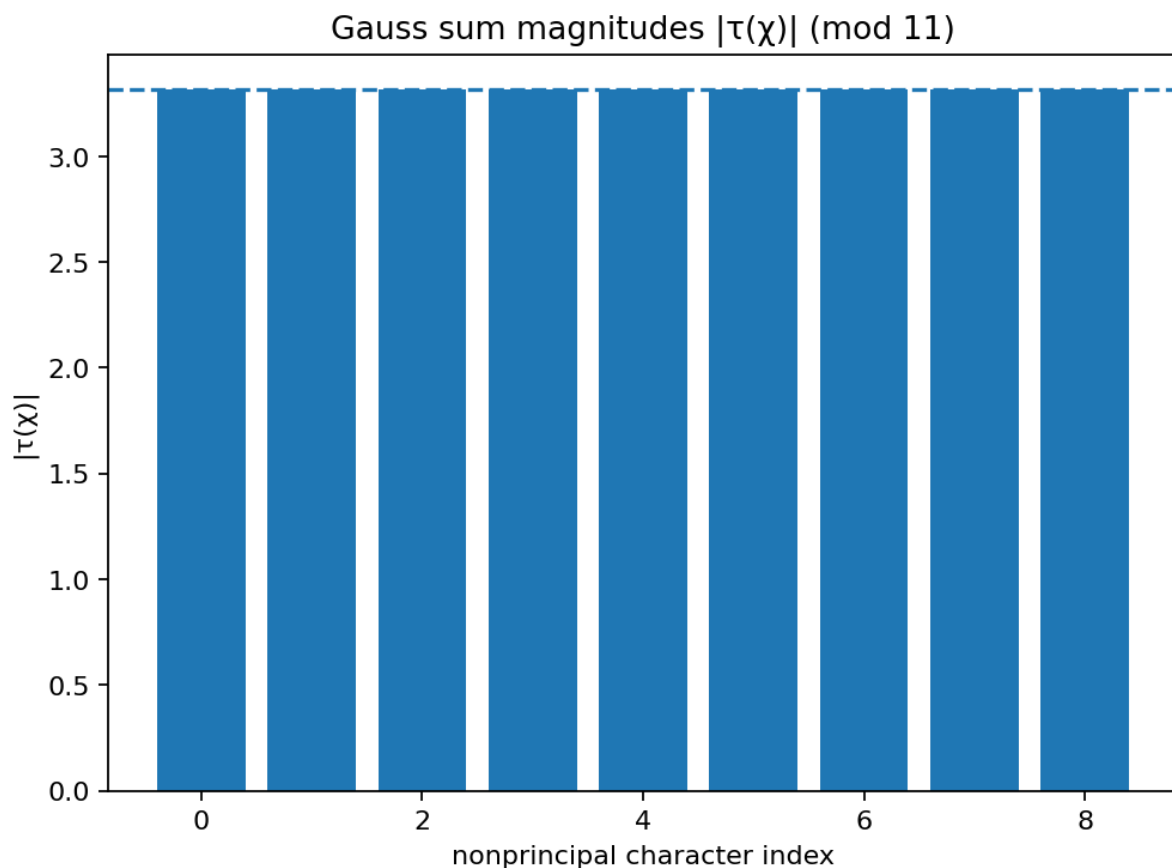
Fig. 29: E109 — Gauss sums: magnitude patterns
