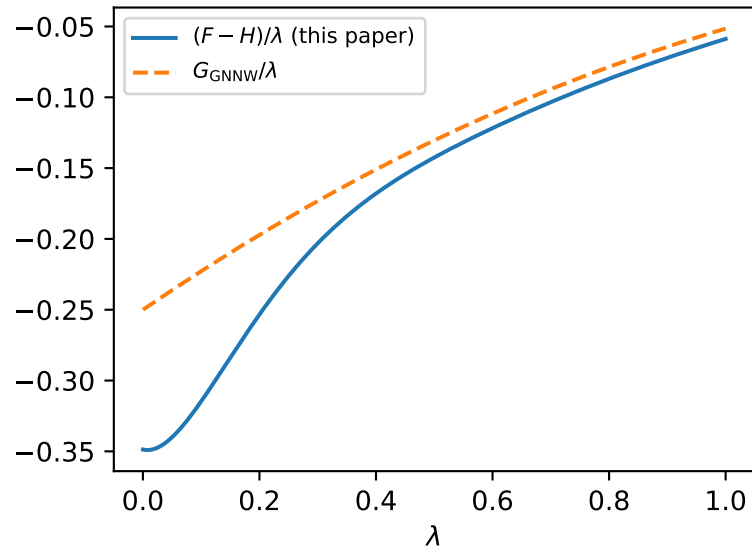
correction to Erdős-Szekeres
