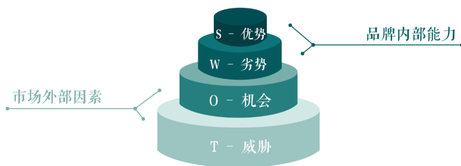
图 10 SWOT 分析法
