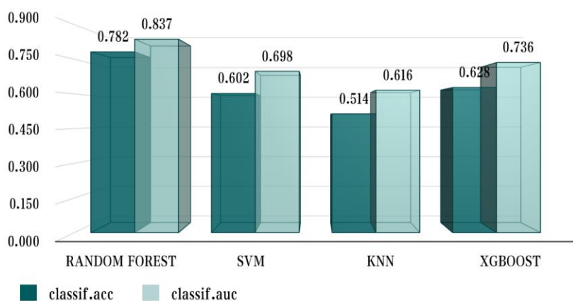
图 54 模型比较
