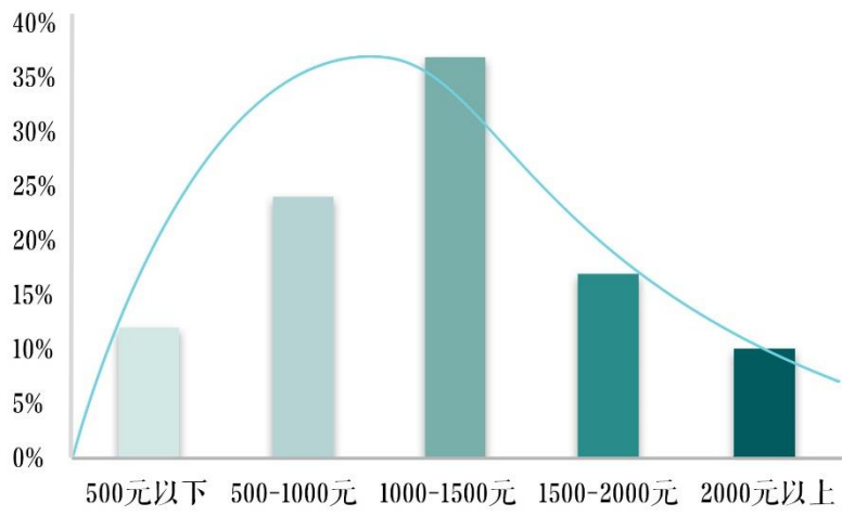
图 71 核密度曲线
