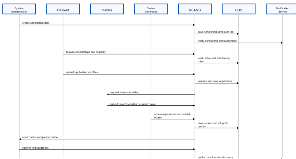
圖八 NSAMS 的系統循序圖
