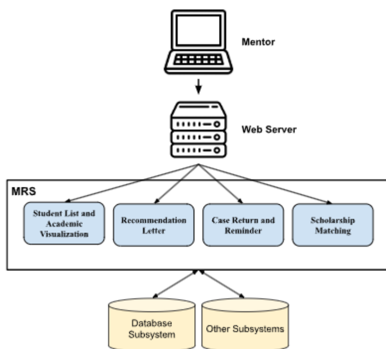
圖十一 MRS 子系統架構圖
