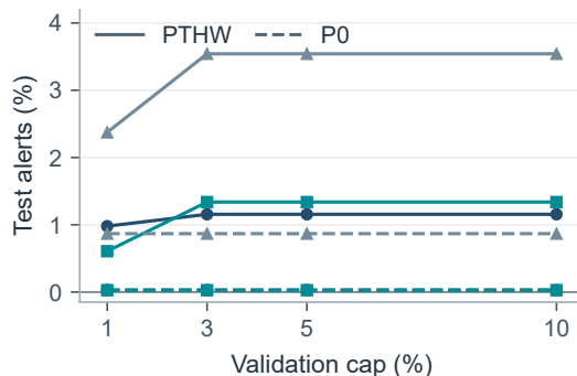
(d) PaySim: workload
