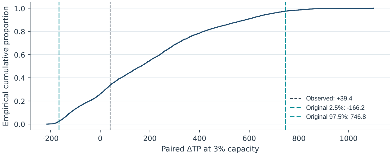
PaySim · Fold 3 · PTHW = PTH · LightGBM · Platt scores
