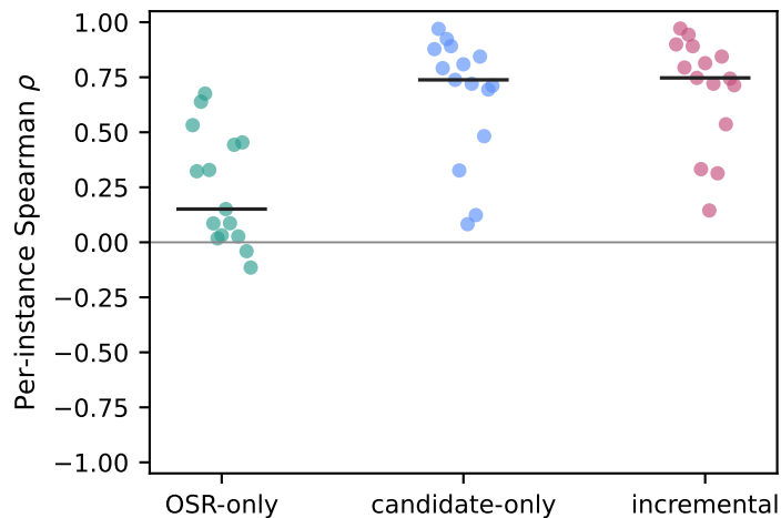
(d) Score vs 20-step decrease 15 instances, 16 candidates each
