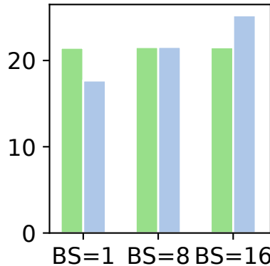
GPT-3-7B-LoRA
