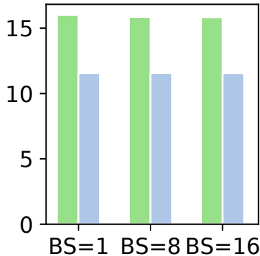
LLaMA-3-8B
