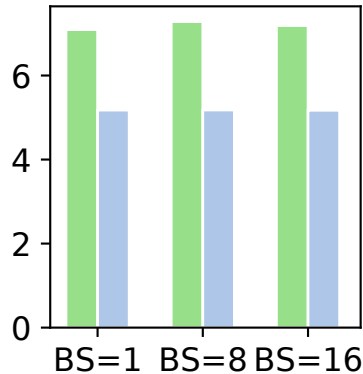
nGPT-1B
