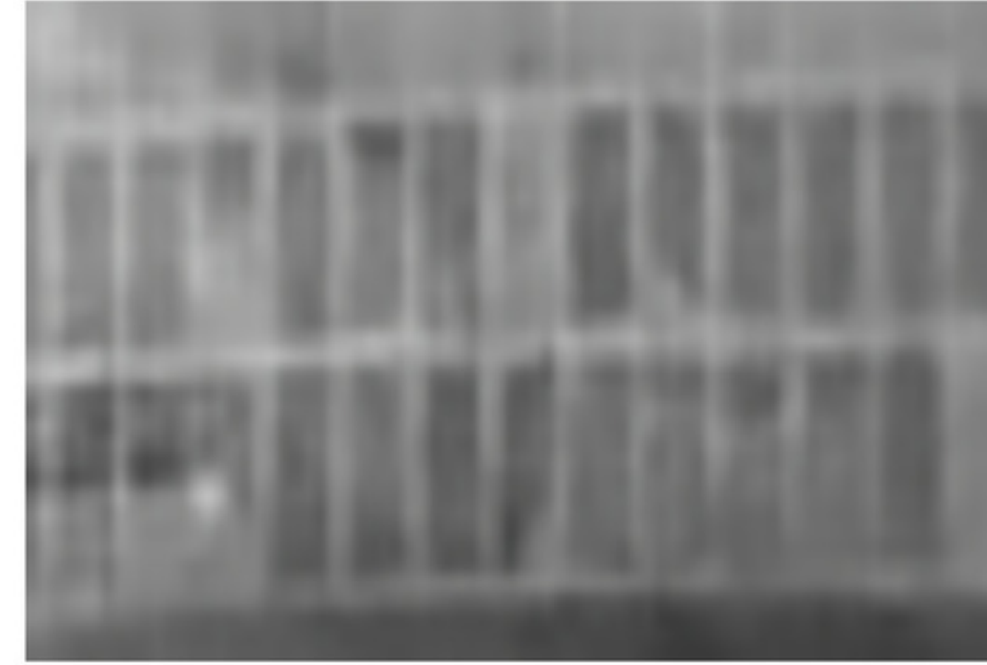
Baseline
