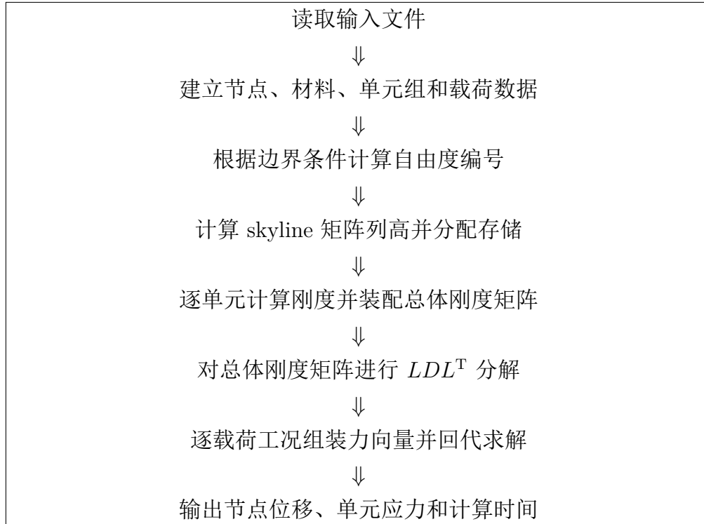
图 1: STAP++ 有限元计算流程
