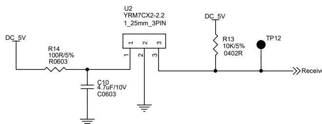
红外接收（基站&主机通讯） 待机1mW Signal_Receive
