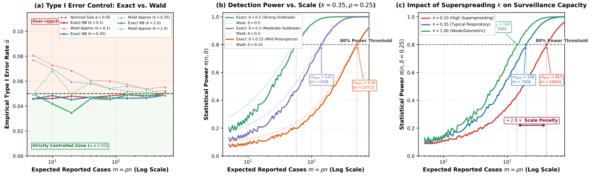
图 2: 早期暴发检验尺度效应、功效边界与超传播惩罚。(a) 一类错误率控制：渐近正态 Wald 检验（虚线）在低病例规模 ( m < 40 ) 且严重超传播 ( k = 0.1 ) 时经验一类错误率最高达 8.1% ( m = 5 , 30,000 次模拟)，系统性高于名义水平；离散精确负二项检验（实线）在全样本网格上严格控制错误率低于 0.05。(b) 检出功效曲线随备择强度 \delta = R_t - 1 的响应：在 k = 0.35 时，达到 80% 功效所需的期望报告规模由微弱暴发 \delta = 0.15 的 m = 517.8 ( n = 2071 ) 急剧下降至 \delta = 0.30 的 m = 142.0 ( n = 568 ) 与 \delta = 0.50 的 m = 57.2 ( n = 229 )。(c) 个体超传播离散度 k 的杠杆惩罚：在 \delta = 0.25 增长强度下，达到 80% 检出功效所需的期望病例数从低异质性 k = 1.0 的 m = 142.0 ( n = 568 ) 急剧上升至严重超传播 k = 0.1 的 m = 415.0 ( n = 1660 )，规模需求放大了近 3 倍。标称显著性水平 \alpha = 0.05 ，基准报告率 \rho = 0.25 。
