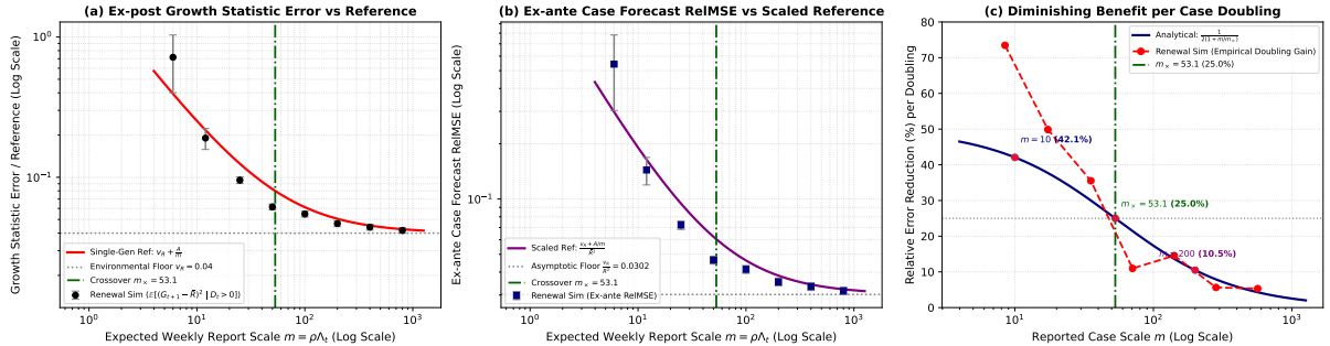
图 3: 更新过程时间序列事后增长统计量与事前单步病例预测误差对照。(a) 事后代理增长统计量均方误差 (黑色散点带 95% 置信区间) 与单代已知基准参照曲线 V(m) = v_R + A/m (红实线, 其中 A = 2.1232, v_R = 0.04 ) 的对照; (b) 事前单步病例预测相对均方误差 (蓝色方块带 95% 置信区间) 与缩放参照曲线 \frac{v_R + A/m}{\bar{R}^2} (紫实线): m \geq 25 段贴合 (参照的 0.75–0.98 倍), m = 6 处为参照的 1.82 倍; (c) 病例规模每翻一倍所带来的相对误差削减百分比: 红圈为更新过程经验翻倍降幅 (事后统计量与事前预测经验降幅严格同一; m < 12 段经验降幅系统性高于解析式, 首点 m = 6 \rightarrow 12 的 73.5% 超出纵轴范围), 深蓝实线为单代参照曲线的解析公式 \frac{1}{2(1+m/m_x)} 。在 m = 10 时, 参照翻倍削减为 42.1%; 在交叉点 m_x = 53.1 处为 25.0%; 越过交叉点后, 在 m = 200 时边际削减迅速衰减至 10.5%。(样本说明: 每规模组共 150 条轨迹 \times 26 个预测起点 = 3,900 点; m = 6 组剔除 D_t = 0 者 3 点, 有效 3,897 点; m = 12 组剔除 1 点, 有效 3,899 点; m \geq 25 各组有效点均为 3,900 点)。
