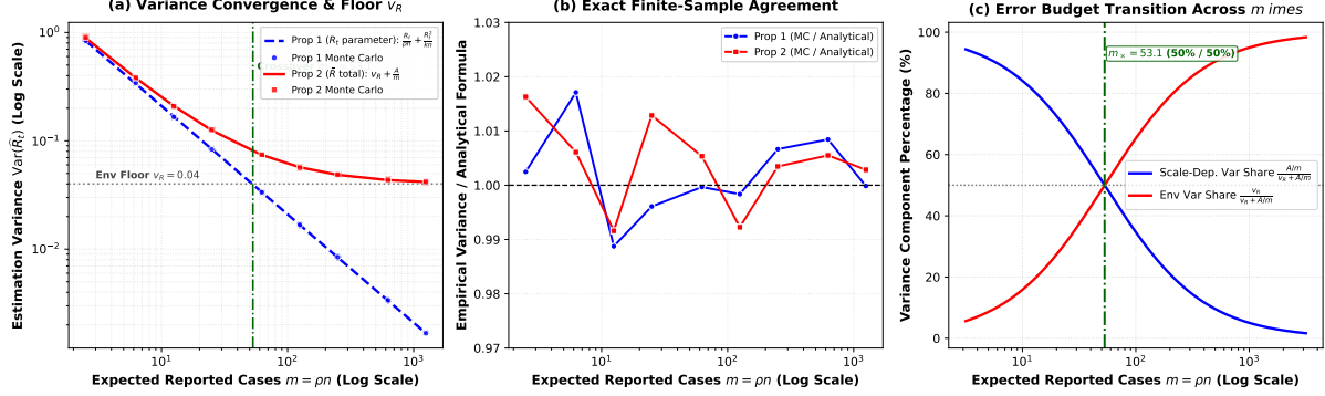
图 1: 理论命题与方差占比交叉点蒙特卡洛验证 (50,000 次模拟, 参数设定 \bar{R} = 1.15, v_R = 0.04, k = 0.35, \rho = 0.25 )。 (a) 当期传播参数测量方差式 (6) (蓝) 与跨期基础水平单期方差式 (7) (红) 随期望报告病例数 m = \rho n 的双对数衰减曲线, 数值模拟散点与理论解析曲线一致, 清楚展现环境方差底板 v_R = 0.04 ; (b) 经验方差与理论推导公式的比值在本次参数网格下处于 0.988–1.017 之间, 有限样本模拟值接近解析值; (c) 误差预算动态演变: 在交叉点 m_{\times} = 53.1 处, 病例规模相关方差与环境扰动各占 50%, 展现了主要误差来源的平滑交接。
