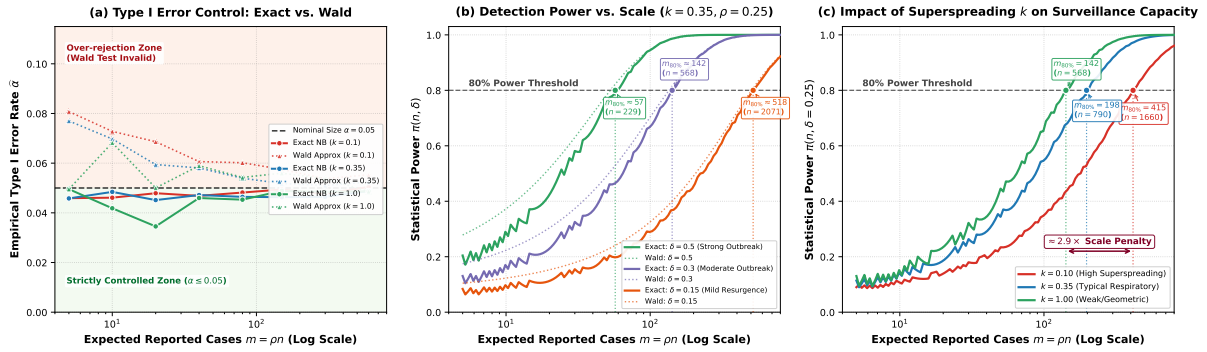
图 2: 当期超临界增长判定检验功效与有限样本性质验证 (名义水平 \alpha = 0.05 , 基准 \rho = 0.25 )。 (a) 第一类错误率 (Size) 控制: 渐近正态 Wald 检验 (虚线) 在低病例规模 ( m < 40 ) 且严重超传播 ( k = 0.1 ) 时经验一类错误率最高达 8.1% ( m = 5 , 30,000 次模拟), 系统性高于名义水平, 而精确负二项非随机化检验 (实线) 在全样本网格上严格控制错误率低于 0.05; (b) 检出功效曲线随择强度 \delta = R_t - 1 的提升, 当 k = 0.35 时, 达到 80% 功效所需的期望报告规模由 \delta = 0.15 的 m = 517.8 ( n = 2071 ) 下降至 \delta = 0.30 的 m = 142.0 ( n = 568 ) 与 \delta = 0.50 的 m = 57.2 ( n = 229 ); (c) 个体超传播离散度 k 的冲击: 在 \delta = 0.25 增长强度下, 达到 80% 检出功效所需的期望病例数从低异质性 k = 1.0 的 m = 142.0 ( n = 568 ) 暴增至严重超传播 k = 0.1 的 m = 415.0 ( n = 1660 ), 需求放大了近 3 倍。
