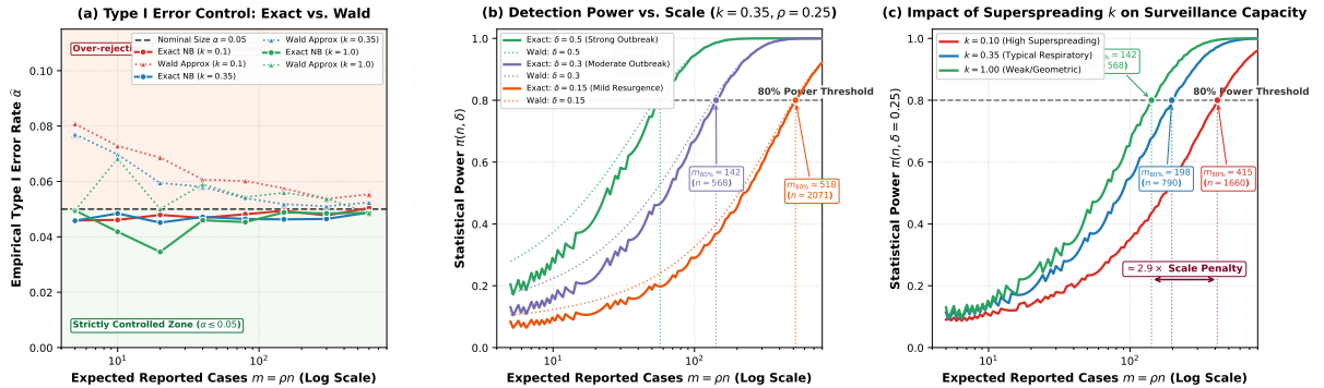
图 2: 早期暴发检验尺度效应、功效边界与超传播惩罚。(a) 一类错误率控制：渐近正态 Wald 检验（虚线）在低病例规模 ( m < 40 ) 且严重超传播 ( k = 0.1 ) 时经验一类错误率最高达 8.1% ( m = 5 , 30,000 次模拟)，系统性高于名义水平；离散精确负二项检验（实线）在全样本网格上严格控制错误率低于 0.05。(b) 检出功效曲线随备择强度 \delta = R_t - 1 的响应：在 k = 0.35 时，达到 80% 功效所需的期望报告规模由微弱暴发 \delta = 0.15 的 m = 517.8 ( n = 2071 ) 急剧下降至 \delta = 0.30 的 m = 142.0 ( n = 568 ) 与 \delta = 0.50 的 m = 57.2 ( n = 229 )。(c) 个体超传播离散度 k 的杠杆惩罚：在 \delta = 0.25 增长强度下，达到 80% 检出功效所需的期望病例数从低异质性 k = 1.0 的 m = 142.0 ( n = 568 ) 急剧上升至严重超传播 k = 0.1 的 m = 415.0 ( n = 1660 )，规模需求放大了近 3 倍。标称显著性水平 \alpha = 0.05 ，基准报告率 \rho = 0.25 。
