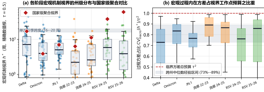
图 4: NB2 模型内机制视界的州级分布、国家级聚合值对比与方差主导比率。(a) 各流行阶段州级辖区机制视界 h^* 的箱线图与散点分布, 红色菱形为国家级视界; (b) 视界临界点处的宏观过程方差主导比率 CV_{macro}^2(h^*)/\tau^2 , 跨阶段中位数达 0.73–0.89。
