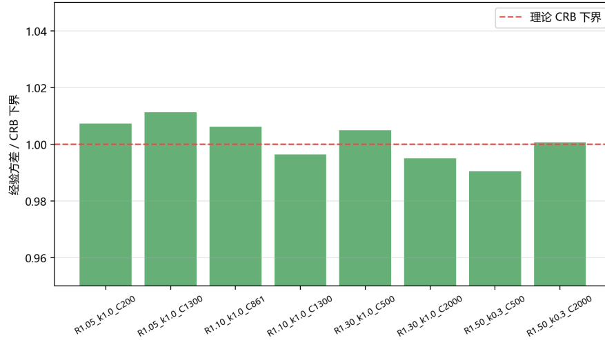
图 4 负二项分支似然下的 Cramér–Rao 辨识界模拟验证。展示在定理 4 的固定观测设定下，不同参数 ( R \in \{1.05, 1.10, 1.30, 1.50\} , k \in \{0.3, 1.0\} ，含单位信噪比基准 C = 861 与 80% 功效工作点 C = 1,300 等) 下极大似然估计量 (MLE) 经验抽样方差与 CRB 基准之比 (该比值围绕 1.000 波动，区间 0.9904–1.0112，虚线为理论下界)，证实了数值实验的精确性。
