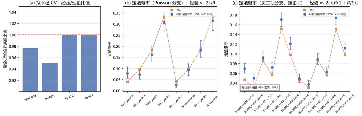
图 3 反射正则化辅助扩散平稳密度与有限种群首达概率的近临界模拟验证。(a) 平稳密度 \pi(x) \propto x^{-1} \exp(c_1 x - c_2 x^2) ( N = 2000 ) 的经验/理论变异系数比值: 近临界 (\varepsilon, R) = (0.005, 1.005), (0.01, 1.01) 为 0.976 与 0.950, 超临界 (0.2, 1.2), (0.4, 1.4) 为 0.9995 与 0.9991。(b) Poisson 分支定殖概率 (8 组, 每组 400 次重复) 与理论 2\varepsilon/R 的对照, 7/8 组落入 95% Beta 区间。(c) 推论 2 负二项设定 (12 组, k \in \{0.5, 1.0\} , 每组 2,500 次重复): 有限种群首达概率与连续扩散代理 2\varepsilon/[R(1 + R/k)] 的对照; k 抑制方向与经验一致, 但因有限种群首达规模 ( \lceil 0.05N \rceil ) 与无界种群终极逃逸灭绝的定义差异, 一阶理论值仅 5/12 落入经验区间且整体偏低 ( N = 500 时经验/理论达 1.07–1.61), 故推论 2 仅作方向性验证。数据来源 verify_t3.json , 重建自 scripts_v2/sim_verify_t3.py 。
