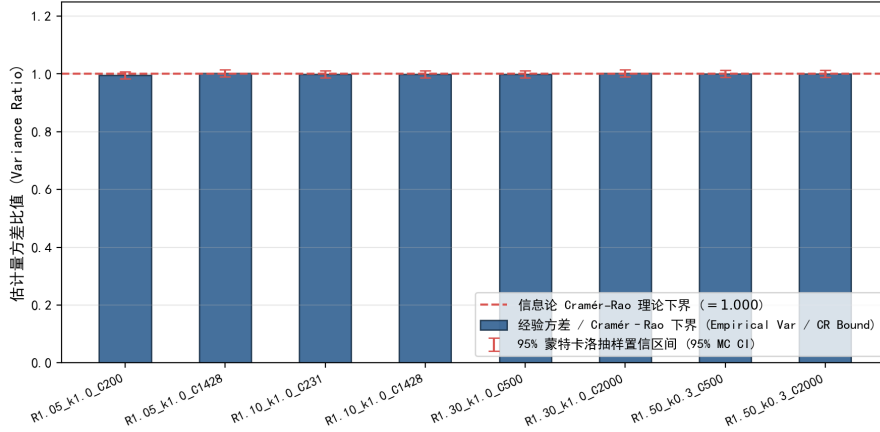
图 4: 定理 4 负二项子代分布下最大似然估计量达到 Cramér-Rao 渐近有效界验证
