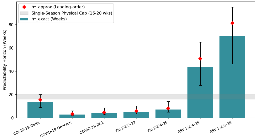
图 5 美国三大呼吸道传染病典型阶段的可预测视界对比。展示各阶段理论预测视界精确根 h_{exact}^* （深青色柱高代表周数，误差棒代表 95% 参数 Bootstrap 置信区间）与一阶闭式渐近基准 h_{approx}^* （橙红菱形点）。灰色虚线与浅灰阴影带标示呼吸道感染病单流行季自然物理跨度（16–20 周）。各阶段详细代数视界与数值对照参见表 2。
