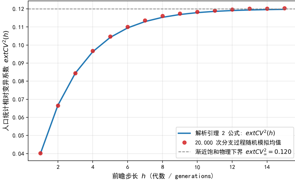
图 2：分支过程变异系数 \text{extCV}^2(h) 的理论推导与随机模拟吻合验证
