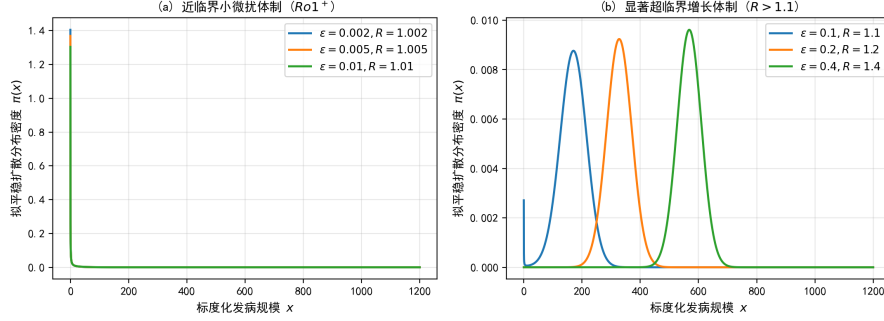
图 3: 定理 3 有限种群近临界拟平稳扩散密度 \pi(x) 的相变演化
