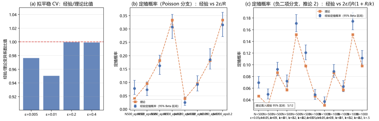
图 3 反射正则化辅助扩散平稳密度与有限种群首达概率的近临界模拟验证。(a) 平稳密度 \pi(x) \propto x^{-1} \exp(c_1 x - c_2 x^2) ( N = 2000 ) 的经验/理论变异系数比值：近临界 (\varepsilon, R) = (0.005, 1.005), (0.01, 1.01) 为 0.976 与 0.950，超临界 (0.2, 1.2), (0.4, 1.4) 为 0.9995 与 0.9991。(b) Poisson 分支定殖概率 (8 组，每组 400 次重复) 与理论 2\varepsilon/R 的对照，7/8 组落入 95% Beta 区间。(c) 推论 2 负二项设定 (12 组， k \in \{0.5, 1.0\} ，每组 2,500 次重复)：有限种群首达概率与连续扩散代理 2\varepsilon/[R(1 + R/k)] 的对照； k 抑制方向与经验一致，但因有限种群首达规模 ( \lceil 0.05N \rceil ) 与无界种群终极逃逸灭绝的定义差异，一阶理论值仅 5/12 落入经验区间且整体偏低 ( N = 500 时经验/理论达 1.07–1.61)，故推论 2 仅作方向性验证。数据来源 verify_t3.json ，重建自 scripts_v2/sim_verify_t3.py 。
