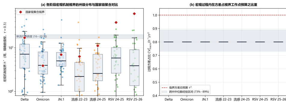
图 4 NB2 模型内机制视界的州级分布、国家级聚合值对比与方差主导比率。 (a) 各流行阶段州级辖区插件式 NB2 模型内机制视界 h^*_{exact} (周, 对数纵轴) 的箱线图与抖动散点分布 (按病原体着色), 红色空心菱形为 51 个州级辖区求和的国家级序列视界。国家级值在七个阶段中的六个高于州级中位数 (唯一例外是 Omicron), 展示空间聚合平滑对机制视界的抬升; (b) 视界临界工作点处的宏观过程方差主导比率 CV^2_{macro}(h^*)/\tau^2 , 跨阶段中位数稳定在 0.73–0.89, 表明宏观过程离散度构成了州级机制视界的核心刚性约束。灰色带标示呼吸道病毒单流行季 16–20 周的自然跨度。
