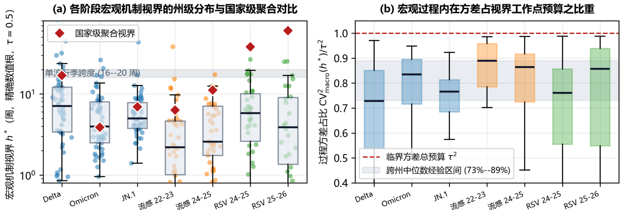
图 4 NB2 模型内机制视界的州级分布、国家级聚合值对比与方差主导比率。(a) 各流行阶段州级辖区插件式 NB2 模型内机制视界 h^*_{\text{exact}} （周，对数纵轴）的箱线图与抖动散点分布（按病原体着色），红色空心菱形为 51 个州级辖区求和的国家级序列视界。国家级值在七个阶段中的六个高于州级中位数（唯一例外是 Omicron），展示空间聚合平滑对机制视界的抬升；(b) 视界临界工作点处的宏观过程方差主导比率 \text{CV}^2_{\text{macro}}(h^*)/\tau^2 ，跨阶段中位数稳定在 0.73–0.89，表明宏观过程离散度构成了州级机制视界的核心刚性约束。灰色带标示呼吸道病毒单流行季 16–20 周的自然跨度。
