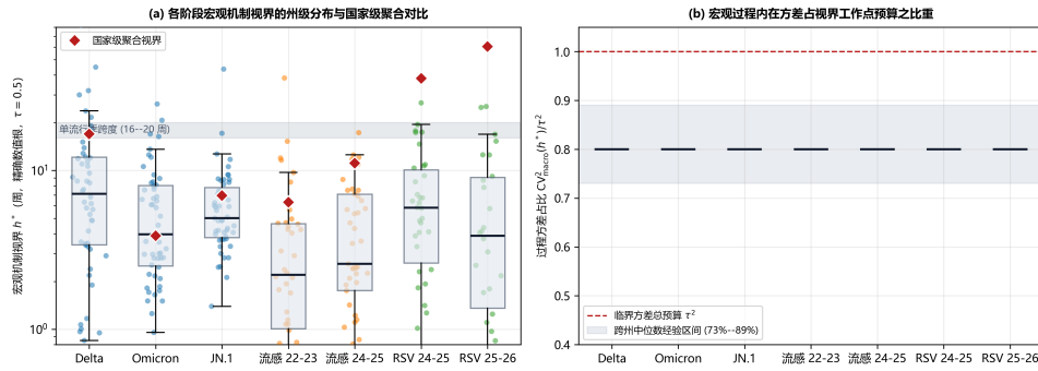
图 4 宏观机制视界的州级分布、国家级聚合值对比与方差主导比率。(a) 各流行阶段州级辖区固定参数 NB2 模型内机制视界 h_{\text{exact}}^* （周，对数纵轴）的箱线图与抖动散点分布（按病原体着色），红色空心菱形为 51 个州级辖区求和的国家级序列视界。国家级值在七个阶段中的六个高于州级中位数（唯一例外是 Omicron），展示空间聚合平滑对机制视界的抬升；(b) 视界临界工作点处的宏观过程方差主导比率 \text{CV}_{\text{macro}}^2(h^*)/\tau^2 ，跨阶段中位数稳定在 0.73–0.89，表明宏观过程离散度构成了州级机制视界的核心刚性约束。灰色带标示呼吸道病毒单流行季 16–20 周的自然跨度。
