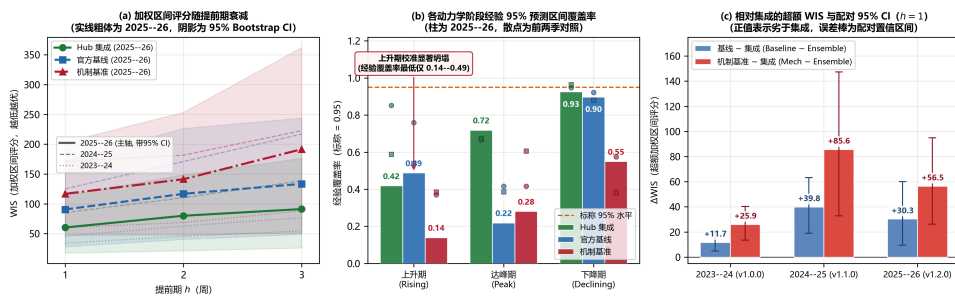
图 5CDC FluSight 三个连续赛季外部审计与动力学阶段分层校准特征。(a) 三个锁定赛季加权区间评分 (WIS) 随提前期 h 的衰减轨迹 (实线粗体为 2025–26 赛季并附 95% Bootstrap CI 阴影带, 虚线与点线为前两季对照), 展示 Hub 集成对官方基线与启发式插件式机制预测器的持续优势; (b) 各动力学阶段经验 95% 预测区间覆盖率 ( h = 1 , 柱状为 2025–26 赛季, 散点为前两季对照, 橙色虚线为标称 95% 水平), 在多个模型—赛季组合中观察到疫情上升期经验覆盖率较低 (在 2025–26 赛季三模型覆盖率为 0.140–0.488, 全三赛季跨度为 0.140–0.852, 见表 7); (c) h = 1 时各模型相对集成的超额 WIS 及配对 95% Bootstrap 置信区间 (三个赛季中, 相对集成的配对 WIS 差置信区间均未跨越 0)。
