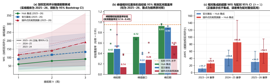
图 5CDC FluSight 三个连续赛季外部审计与峰值相对位置分层校准特征。(a) 三个锁定赛季加权区间评分 (WIS) 随提前期 h 的衰减轨迹 (实线粗体为 2025–26 赛季并附 95% Bootstrap CI 阴影带, 虚线与点线为前两季对照), 展示 Hub 集成对官方基线与启发式插件式机制预测器的持续优势; (b) 各阶段经验 95% 预测区间覆盖率 ( h = 1 , 柱状为 2025–26 赛季, 散点为前两季对照, 橙色虚线为标称 95% 水平), 在多个模型—赛季组合中观察到疫情峰前期经验覆盖率较低 (在 2025–26 赛季三模型覆盖率为 0.140–0.488, 全三赛季跨度为 0.140–0.852, 见表 7); (c) h = 1 时各模型相对集成的超额 WIS 及配对 95% Bootstrap 置信区间 (三个赛季中, 相对集成的配对 WIS 差置信区间均未跨越 0)。
