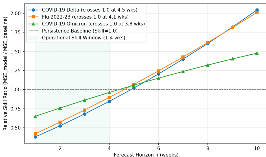
图 7 美国 CDC 真实监测数据滚动样本外预测相对技能衰减曲线。展示 COVID-19 Delta、Omicron 及季节性流感在逐周滚动预测原点下，前瞻步长 h = 1-10 周的相对均方误差技能比 \text{MSE}_{\text{model}}/\text{MSE}_{\text{baseline}} 。在近程（ h \leq 2-4 周）内，动力学模型优于持续性基线（技能比为 0.38–0.89）；在步长超越 4 周后，外生残差迅速膨胀，技能比在 h \approx 3.8-4.6 周穿过 1.0 水平线（灰色虚线），表明实际有效预测时效被压缩至 1–4 周，展现了理论机制上限与经验有效预测时效的双层分析框架。
