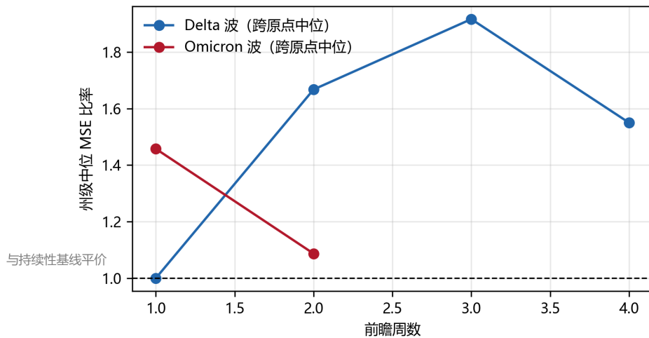
图 7 COVIDhub-ensemble 集成预测的州级技能衰减。 纵轴为跨州中位平方误差比率 SERatio (相对持续性基线), 横轴为前瞻周数, 黑色虚线为与持续性基线平价 (SERatio = 1)。Delta 与 Omicron 两波共 12 个预测原点: 两波的中位平方误差比率均在 1–2 周内越过或逼近平价线, 与本文自设模型给出的业务时效区间一致。
