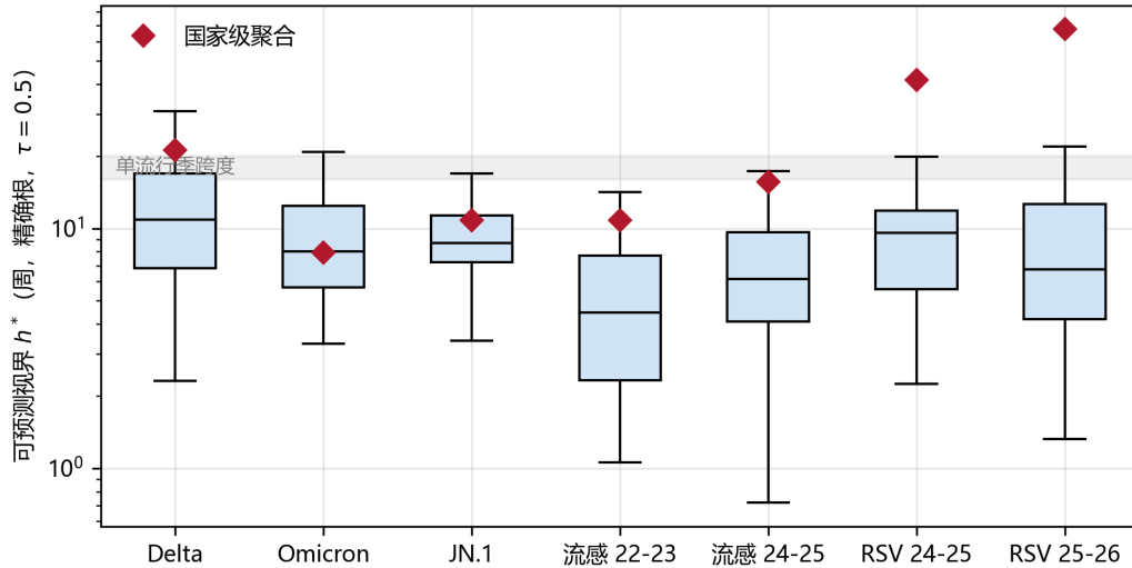
图 6 各阶段机制代理视界的州级分布与国家级聚合值对比。箱线图为州级辖区 h_{\text{exact}}^* （周，对数纵轴）的中位数与四分位距，红色菱形为 51 州求和的国家级序列在同一窗口的视界。国家级值在七个阶段中的六个高于州级中位数（唯一例外是 Omicron，两者基本相等），直观展示聚合平滑对代理视界的抬升及其边界。灰色带标示呼吸道病毒单流行季 16–20 周的自然跨度。
