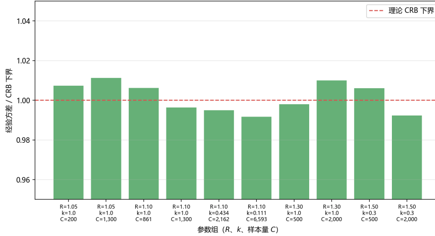
图 4 负二项分支似然下的 Cramér–Rao 辨识界模拟验证。展示在定理 4 的固定观测设定下，居中参照 k = 1.0 与本文实测 k \in \{0.434, 0.111\} 三档、不同 R 与样本量 C 下极大似然估计量 (MLE) 经验抽样方差与 CRB 基准之比 (该比值围绕 1.000 波动，区间 0.9917–1.0112，虚线为理论下界)。含实测 k = 0.434 ( C = 2,162 ) 与 k = 0.111 ( C = 6,593 ) 两个超扩散工作点，证实 CRB 在本文实测离散度区间内仍被 MLE 渐近达到。
