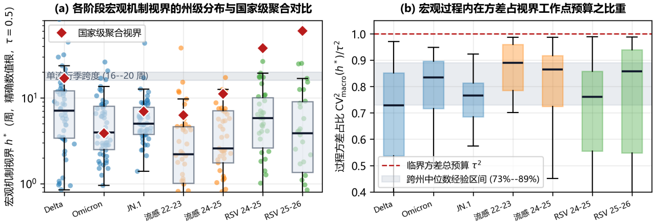
图 4 NB2 模型内机制视界的州级分布、国家级聚合值对比与方差主导比率。(a) 各流行阶段州级辖区插件式 NB2 模型内机制视界 h_{\text{exact}}^* (周，对数纵轴) 的箱线图与抖动散点分布 (按病原体着色)，红色空心菱形为 51 个州级辖区求和的国家级序列视界。国家级值在七个阶段中的六个高于州级中位数 (唯一例外是 Omicron)，展示空间聚合平滑对机制视界的抬升；(b) 视界临界工作点处的宏观过程方差主导比率 CV_{\text{macro}}^2(h^*)/\tau^2 ，跨阶段中位数稳定在 0.73–0.89，表明宏观过程离散度构成了州级机制视界的核心刚性约束。灰色带标示呼吸道病毒单流行季 16–20 周的自然跨度。
