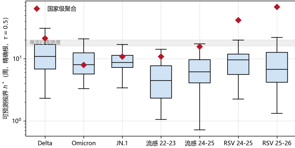
图 6 各阶段机制代理视界的州级分布与国家级聚合值对比。 箱线图为州级辖区 h_{\text{exact}}^* (周, 对数纵轴) 的中位数与四分位距, 红色菱形为 51 州求和的国家级序列在同一窗口的视界。国家级值在七个阶段中的六个高于州级中位数 (唯一例外是 Omicron, 两者基本相等), 直观展示聚合平滑对视界的系统性高估及其边界。灰色带标示呼吸道病毒单流行季 16–20 周的自然跨度。
