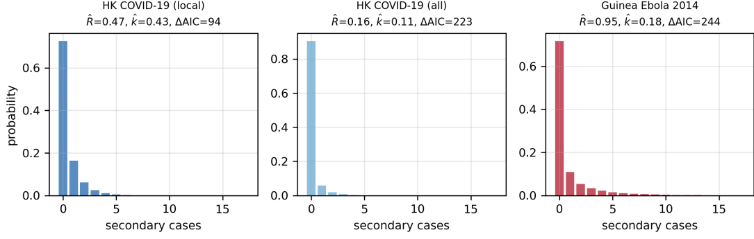
图 5 个体子代分布的负二项拟合。三组传播链数据的拟合负二项概率质量函数与拟合参数 ( \hat{R} , \hat{k} , \Delta\text{AIC} ): 香港 COVID-19 本地子群(左)、香港全队列(中)与几内亚埃博拉(右)。埃博拉的近临界均值 ( \hat{R} = 0.954 ) 与极低离散度 ( \hat{k} = 0.182 ) 共同刻画了强超级传播的传播网络。
