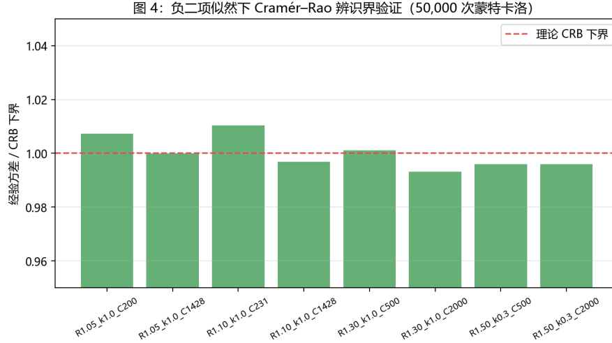
图 4 负二项分支似然下的 Cramér-Rao 辨识界模拟验证。展示在定理 4 的固定观测设定下，不同参数 ( R \in \{1.05, 1.10, 1.30, 1.50\} , k \in \{0.3, 1.0\} , 含关键样本量 231 与模拟工作点 1,428 (对应 80% 功效连续理论值 1,428.7, 向上取整严格最小整数门槛为 1,429) 等) 下极大似然估计量 (MLE) 经验抽样方差与 CRB 基准之比 (该比值围绕 1.000 波动, 区间 0.9931–1.0104, 虚线为理论下界), 证实了数值实验的精确性。
