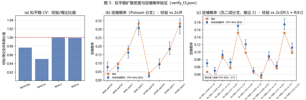
图 3 拟平稳扩散密度与定殖概率的近临界相变模拟验证 (数据来源 verify_t3.json , 重建自 scripts_v2/sim_verify_t3.py )。 (a) 反射正则化辅助扩散平稳密度 \pi(x) \propto x^{-1} \exp(c_1 x - c_2 x^2) 在宿主种群 N = 2000 下的经验/理论变异系数比值 (柱序自左至右按偏离量递增): 临界过渡窗口内 ( |\varepsilon| \leq O(N^{-1/2}) \approx 0.022 ) (\varepsilon, R) \in \{(0.005, 1.005), (0.01, 1.01)\} 为 0.976 与 0.950, 超临界区 (\varepsilon, R) \in \{(0.2, 1.2), (0.4, 1.4)\} 为 0.9995 与 0.9991。 (b) 单种子定殖概率的 Poisson 分支 Galton–Watson 模拟 (8 组, 每组 400 次重复) 与理论 2\varepsilon/R 的对照, 7/8 组的理论值落入经验 95% Beta 区间。 (c) 有限种群首达概率与连续扩散建群概率代理比较 (推论 2 设定, 12 组, k \in \{0.5, 1.0\} , 每组 2,500 次重复): 展示有限种群首达概率与连续扩散代理 2\varepsilon/[R(1 + R/k)] (它与式 (18) 的离散母函数展开在近临界 R \rightarrow 1^+ 处领先阶等价) 的对照; k 抑制方向与经验一致, 但由于有限种群首达有限规模 ( \lceil 0.05N \rceil ) 与无界种群终极逃逸灭绝的截断定义差异, 一阶理论值仅 5/12 落入经验 95% Beta 区间且整体偏低 ( N = 500 时经验/理论达 1.07–1.61), 故推论 2 仅作过度离散负向抑制的方向性验证。
